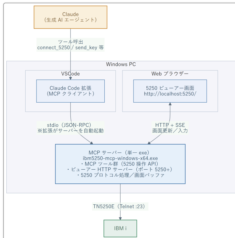
図 1.2-1 システム構成 (Claude / VSCode / ブラウザー / IBM i の関係)
