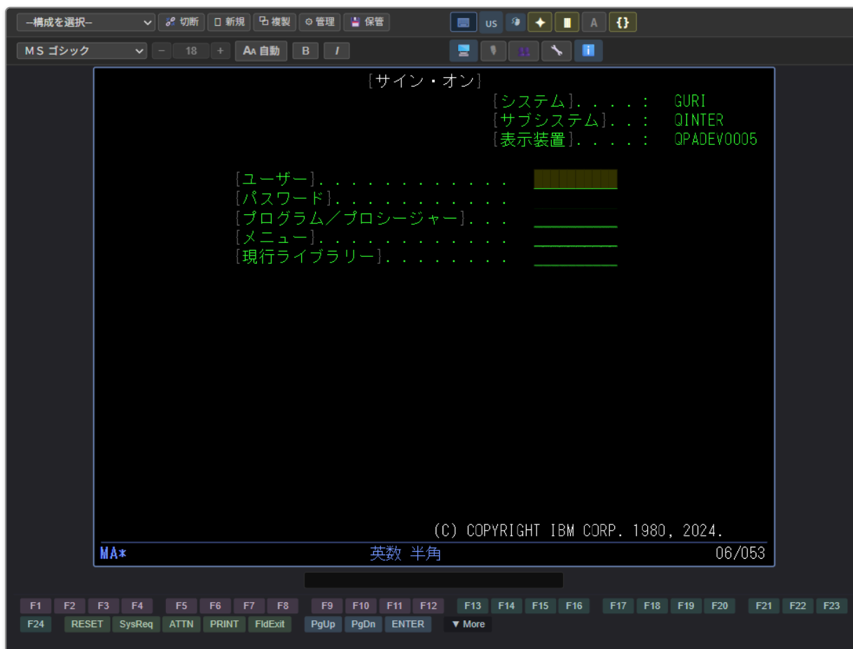
図 3.1-1 サインオン画面
