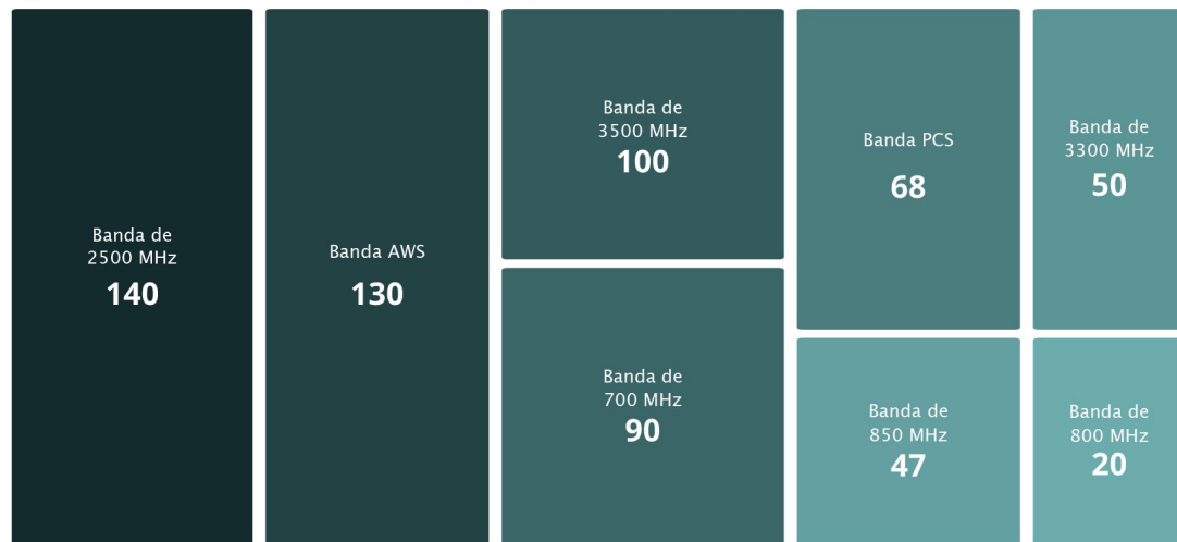
Figura C.1. Espectro radioeléctrico (MHz) asignado por banda de frecuencia
