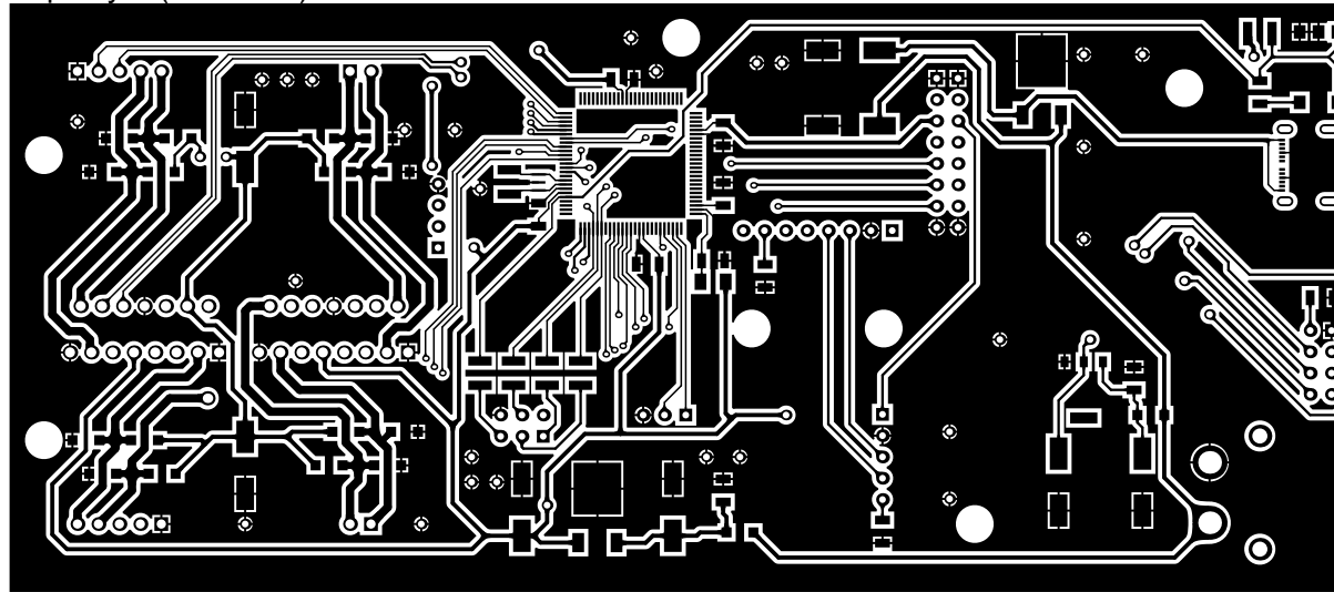
Top Layer (Scale 1:1)
