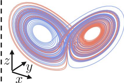
Lorenz
