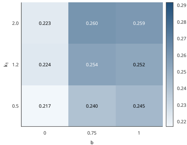
MAP do BM25 por (k1, b)
