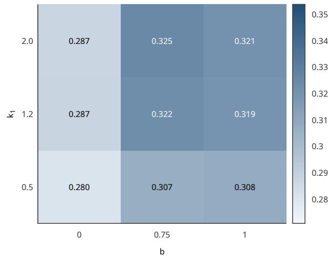
NDCG@10 do BM25 por (k1, b)
