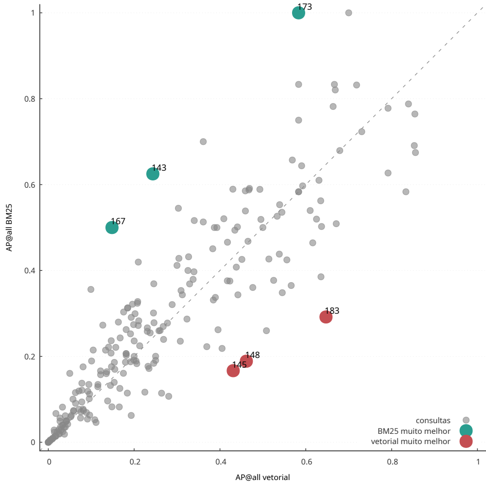
AP@all por consulta, stopwords+stemming (BM25 k1=1.2, b=0.75)
