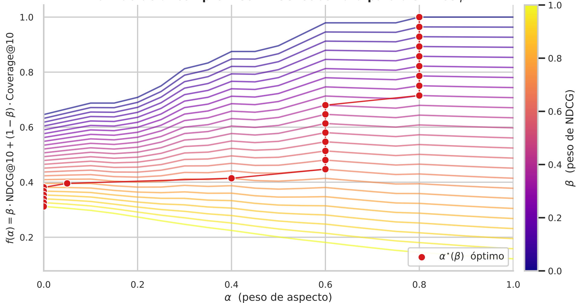
Barrido de \alpha : compromiso NDCG-Cobertura para distintos \beta
