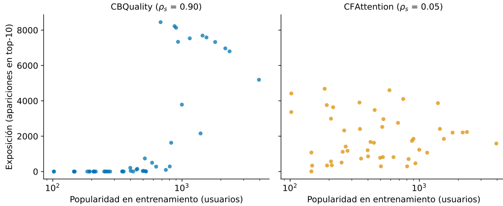
Figura 5.7: Exposición de cada pueblo en función de su popularidad en entrenamiento (escala logarítmica) para las dos ramas del híbrido, con la correlación de Spearman correspondiente. CBQuality exhibe un umbral de popularidad; CFAttention es prácticamente insensible a ella.
