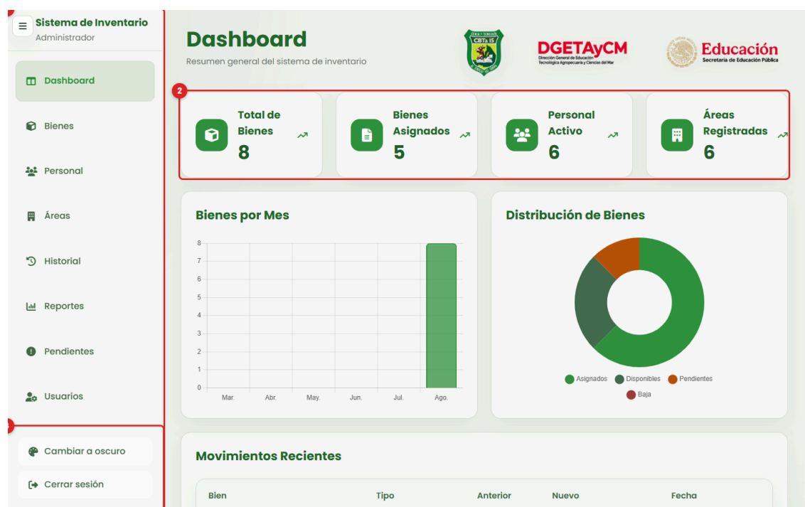
Panel principal: (1) menú lateral, (2) indicadores, (3) tema y cierre de sesión
