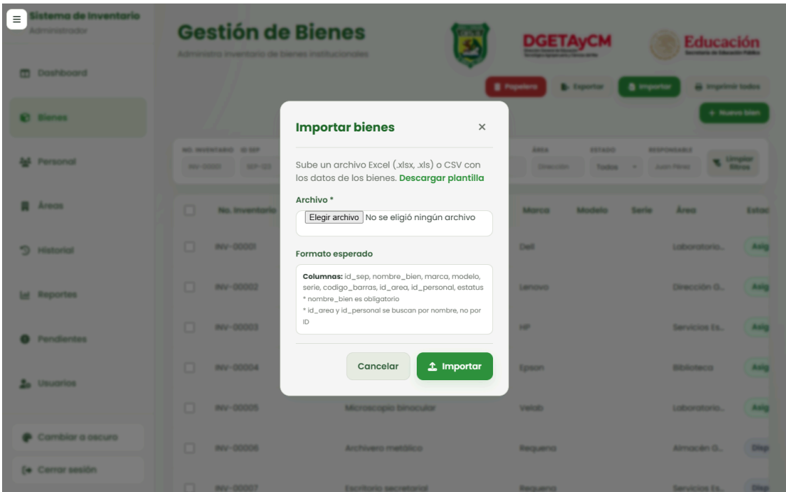
Ventana de importación de bienes
