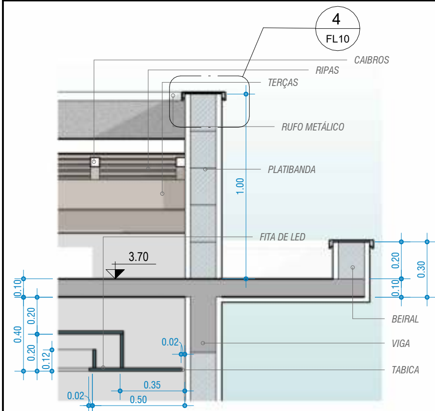
DET. 1 - CORTE 1. SANCA E PLATIBANDA
