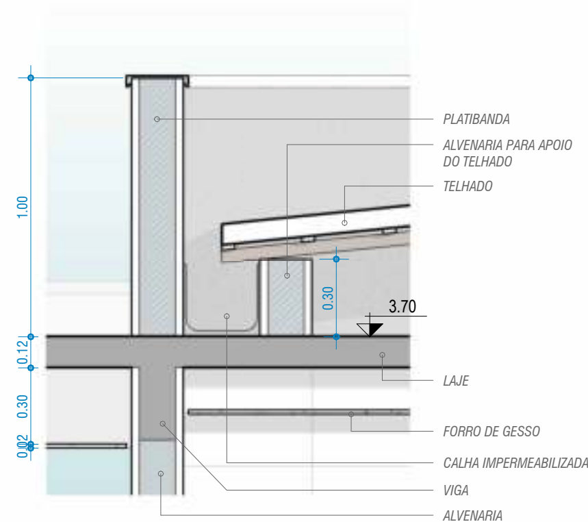
DET. 3 - CORTE 3. CALHA
