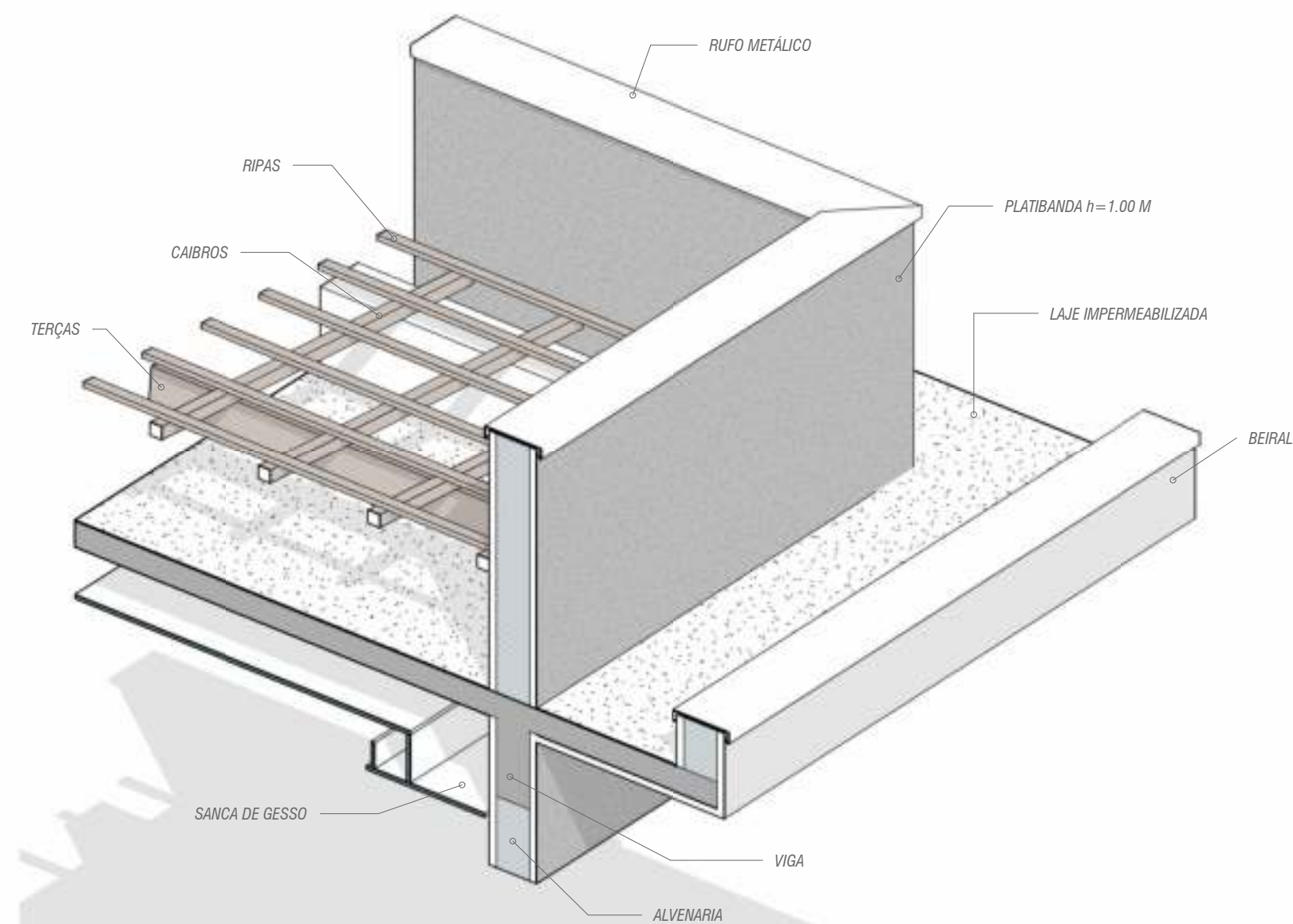
ISOMÉTRICO SANCA E PLATIBANDA
