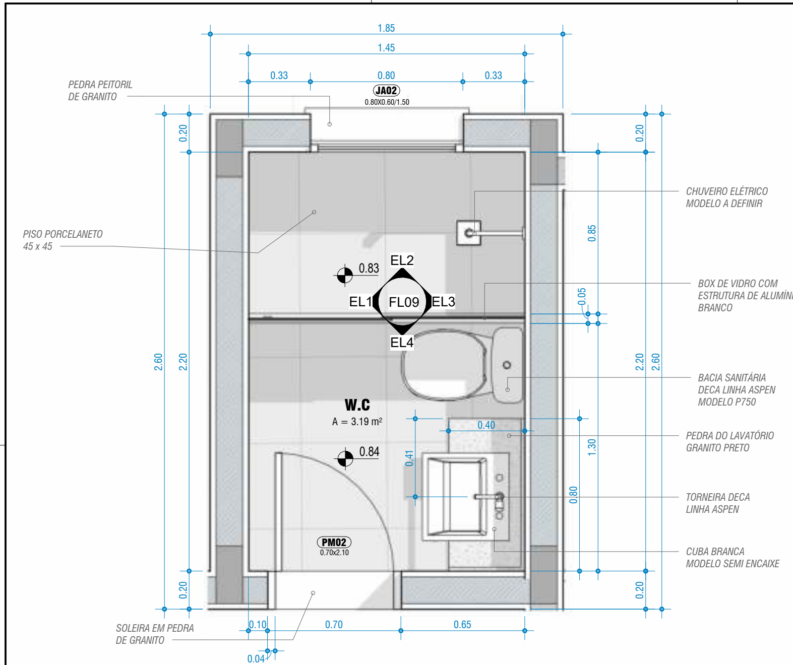
DET. B - PLANTA DETALHE W.C
