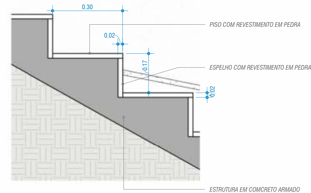
DET. 5 - CORTE 5. ESCADA
