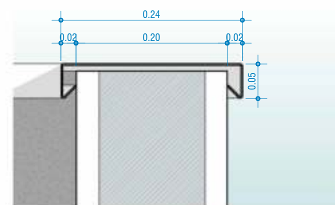
DET. 4 - CORTE 4. RUFO METÁLICO
