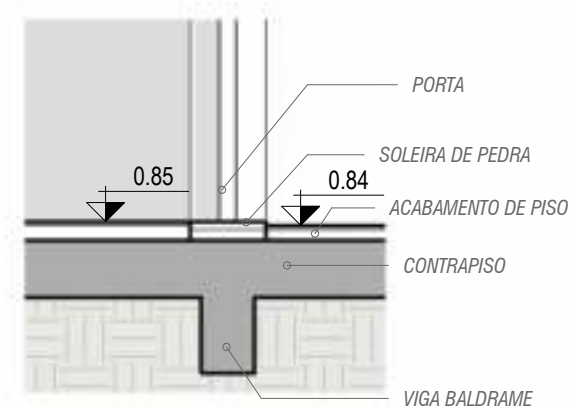
DET. 2 - CORTE 2. - SOLEIRAS
