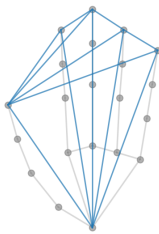
Figura 3. Categorias dos 60 atributos extraídos por mão. (a) 21 distâncias entre articulações, (b) 15 ângulos articulares codificados como par ( \sin , \cos ), (c) 5 atributos de curvatura baseados na diferença em z entre ponta e base de cada dedo, (d) 4 atributos da orientação 3D da palma (pitch e yaw do vetor normal, em \sin/\cos ).
