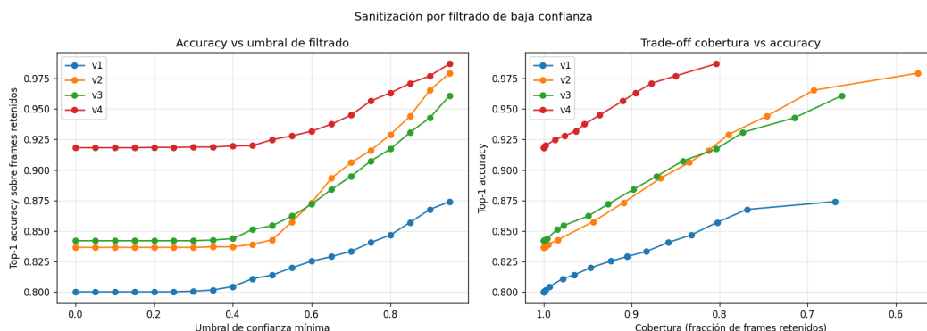
Figura 4. Sanitização por confiança. (Esquerda) acurácia em função do limiar de confiança mínima. (Direita) trade-off entre cobertura e acurácia. v4 oferece a melhor fronteira de Pareto.
