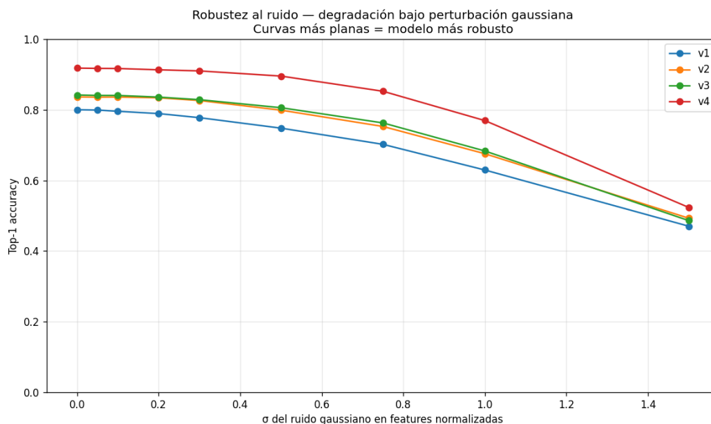
Figura 3. Degradação da acurácia top-1 sob ruído gaussiano aplicado às features normalizadas. Curvas mais planas indicam modelos mais robustos. v4 mantém vantagem estável sobre os demais em todos os níveis de ruído testados.
