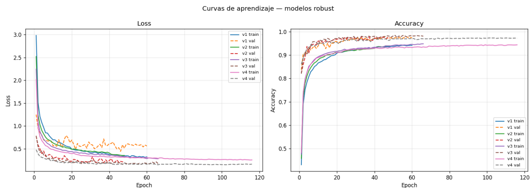
Figura 2. Curvas de loss e accuracy por época para os quatro modelos robustos. v4 (azul-violeta) treina por mais épocas devido ao maior volume de dados (~38 mil amostras de operador vs. ~6 mil em v1), mas converge para val_accuracy superior e mais estável.
