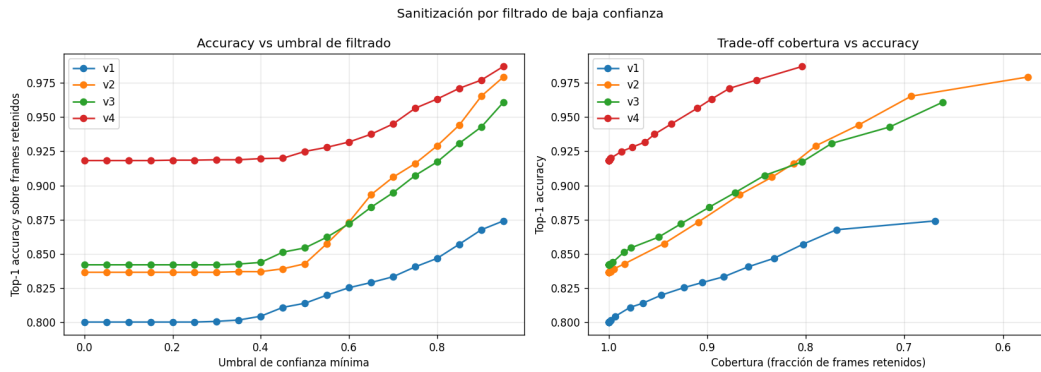
Figura 8. Sanitização por confiança. (Esquerda) acurácia em função do limiar de confiança mínima. (Direita) trade-off entre cobertura e acurácia. v4 oferece a melhor fronteira de Pareto.
