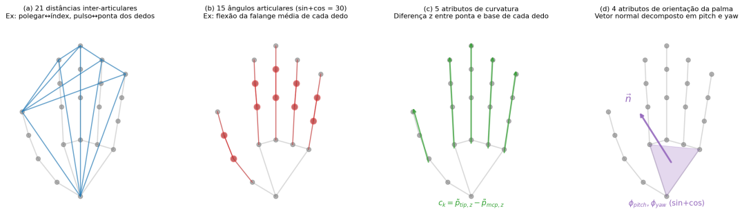
Figura 3. Categorias dos 60 atributos extraídos por mão. (a) 21 distâncias entre articulações, (b) 15 ângulos articulares codificados como par (sin, cos), (c) 5 atributos de curvatura baseados na diferença em z entre ponta e base de cada dedo, (d) 4 atributos da orientação 3D da palma (pitch e yaw do vetor normal, em sin/cos).
