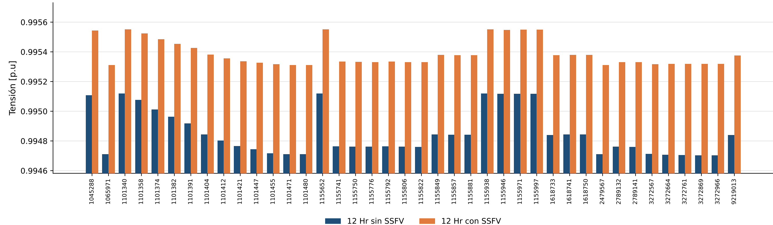
Tensión en nodos a las 12 Horas
