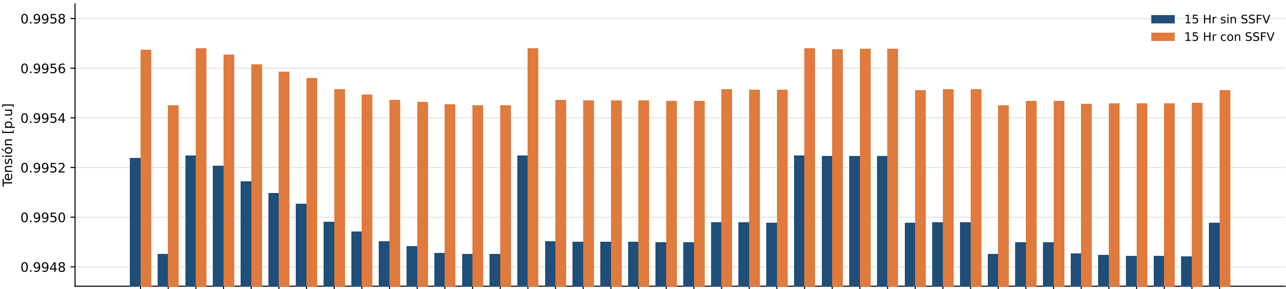
Figura 8. Tensiones en los nodos afectados por el proyecto Mas X Menos sede Guarín 120 kW a las 3 pm
