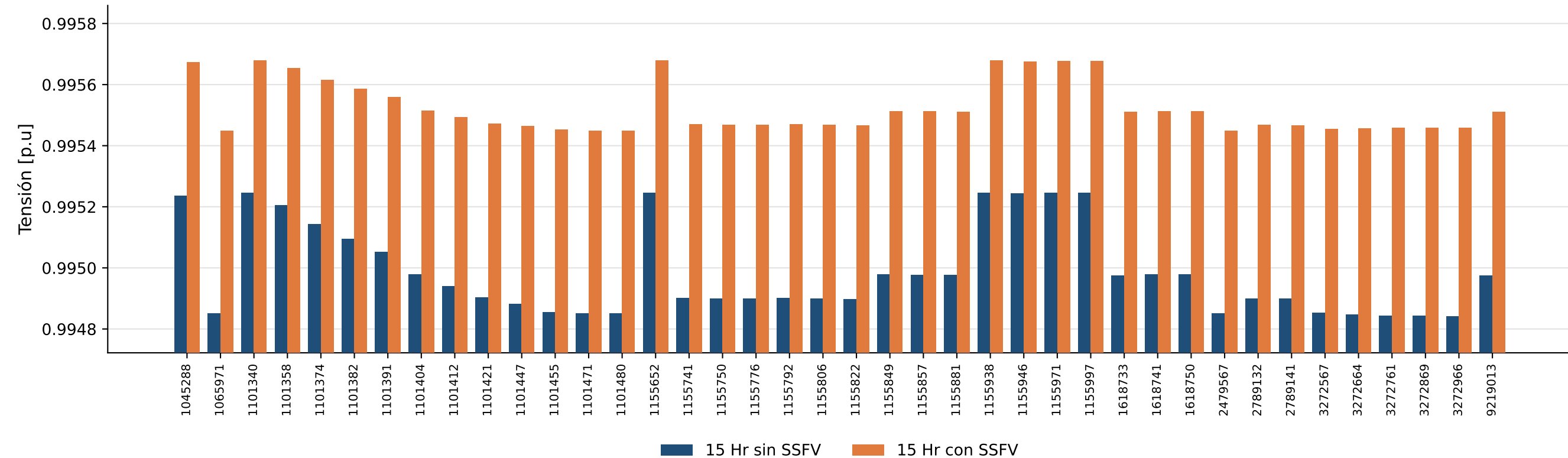
Tensión en nodos a las 15 Horas
