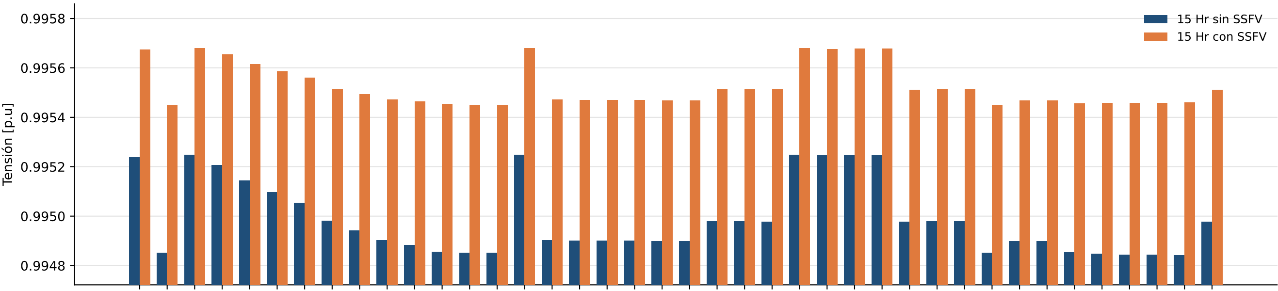
Tensión en nodos a las 15 Horas
