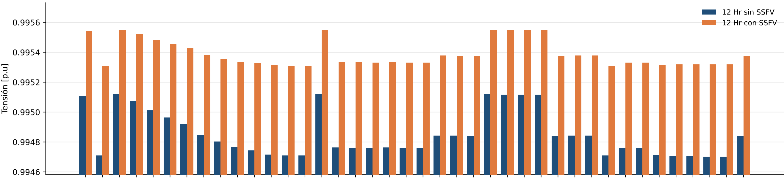
Figura 7. Tensiones en los nodos afectados por el proyecto Mas X Menos sede Guarín 120 kW a las 12 pm
