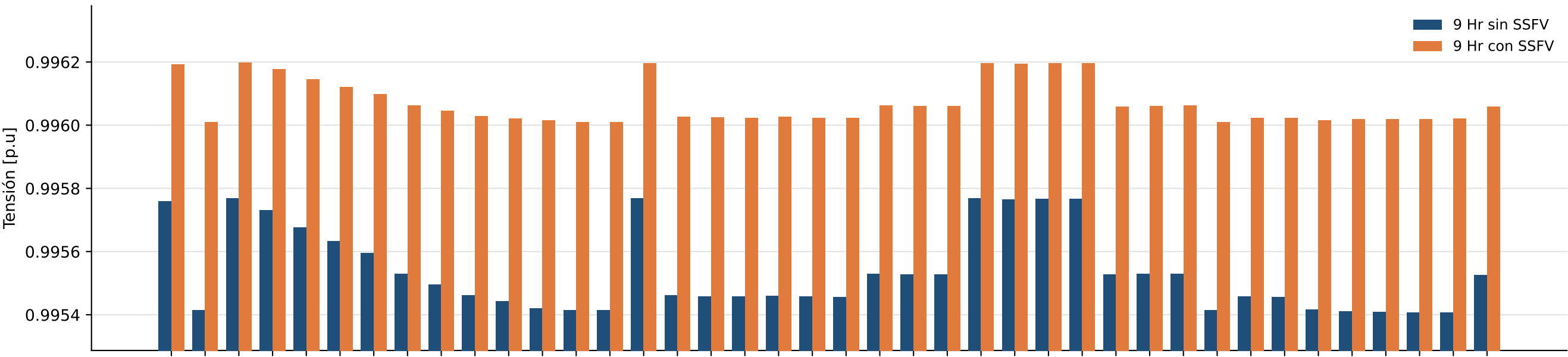
Figura 6. Tensiones en los nodos afectados por el proyecto Mas X Menos sede Guarín 120 kW a las 9 am
