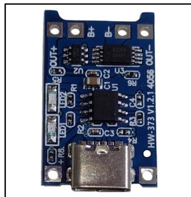
Figura 5 – Módulo TP4056.
