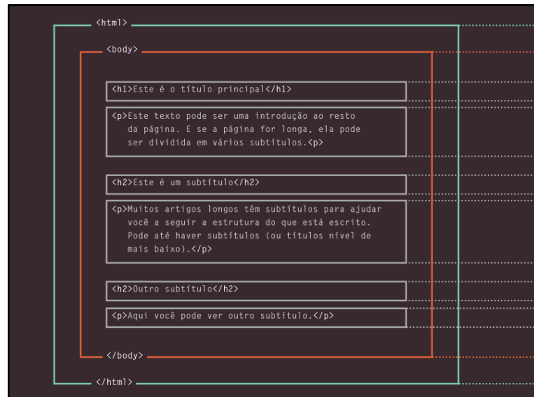
Figura 15 – Exemplo de tags de abertura e de fechamento.
