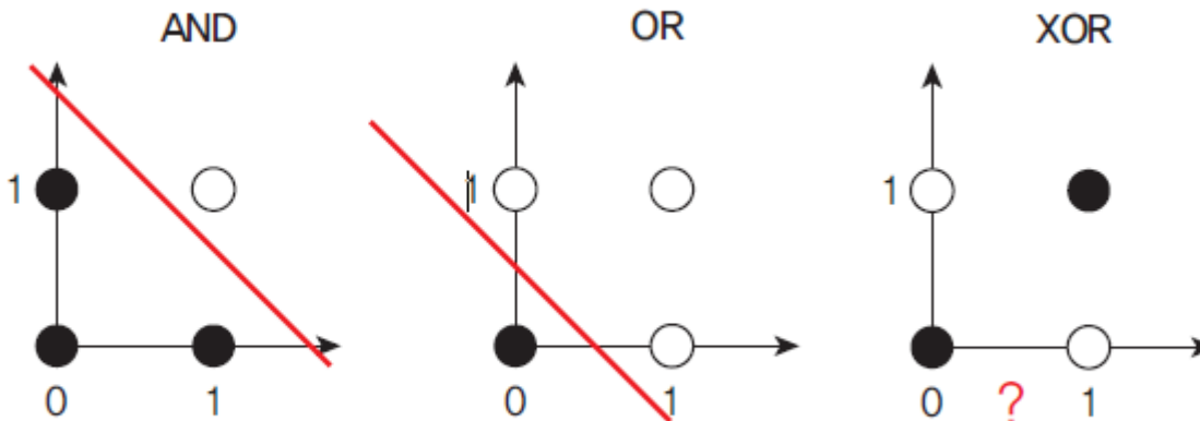
선형 분리 가능한 문제
