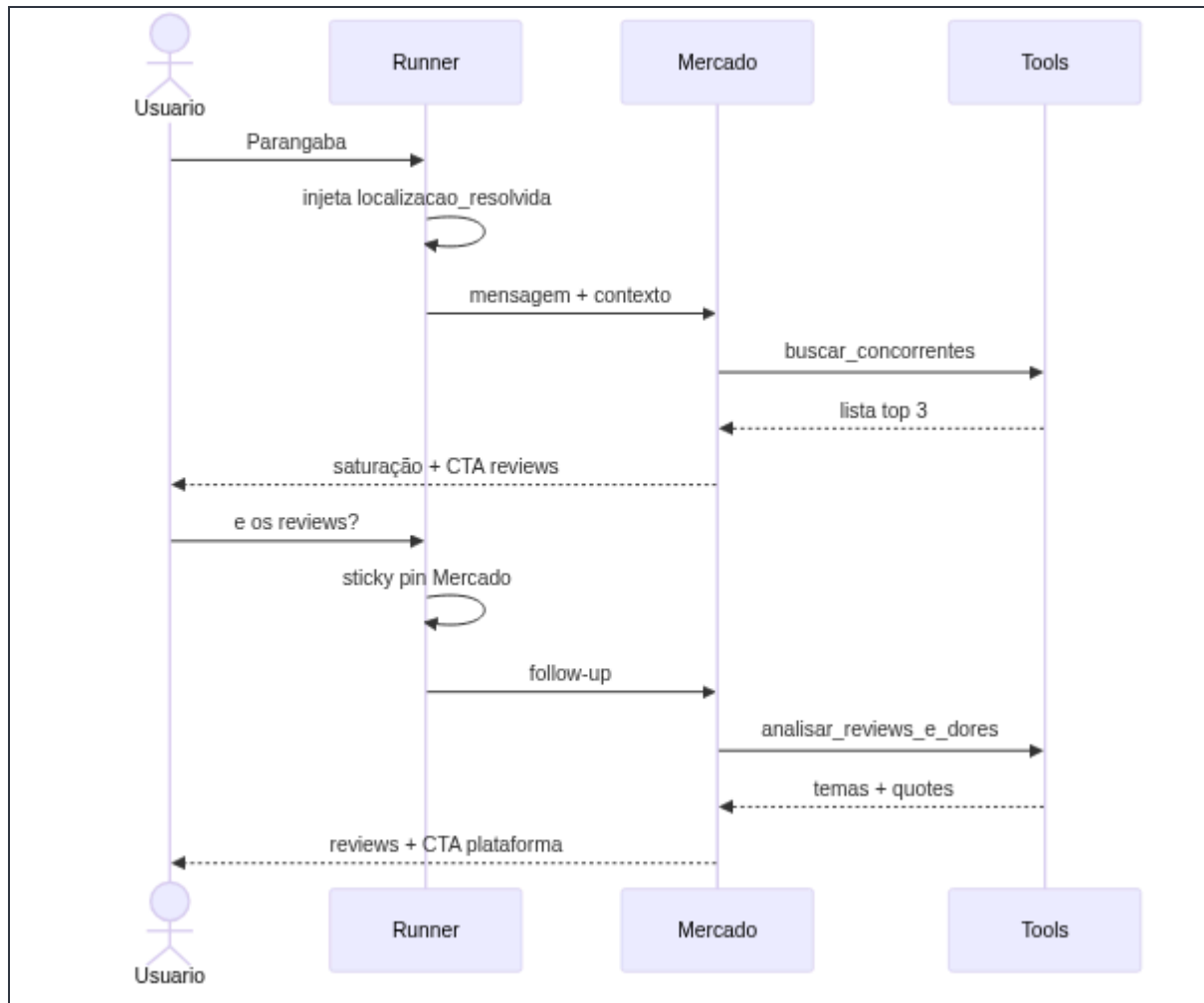
Sequência alvo pós-melhorias
