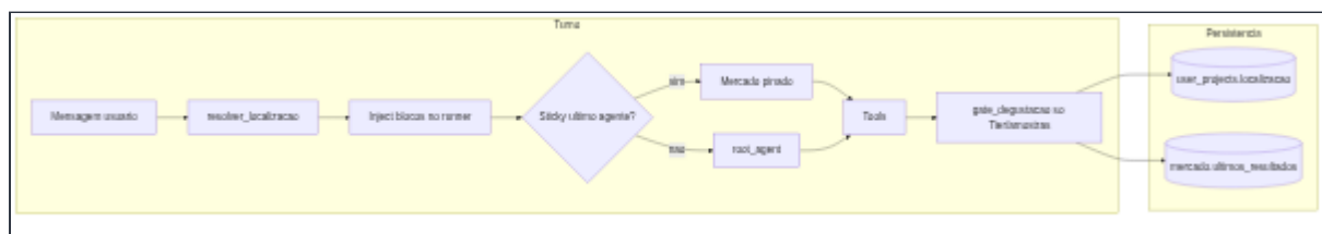
Arquitetura canônica do turno
