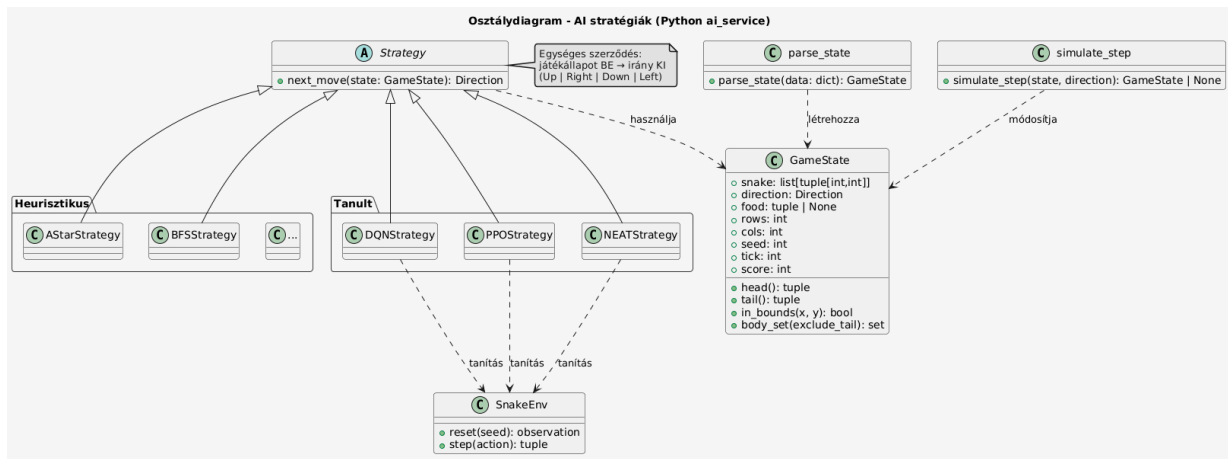
3.4. ábra – AI osztálydiagram: a közös Strategy interfész, a heurisztikus és tanult implementációk, valamint a GameState és SnakeEnv kapcsolata.
