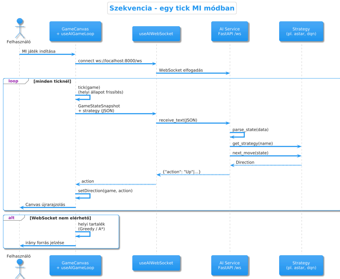
3.5. ábra – Szekvencia: MI játék indítása, WebSocket kapcsolat, majd tickenként állapot küldése → stratégia → irány vissza; ha a WebSocket nem elérhető, helyi tartalék lép életbe.
