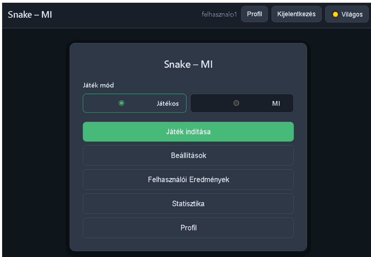
6.2. ábra – Főmenü (MainMenu): játékmód gombok a módhoz, gombok a többi nézethez és a játék indításához.
