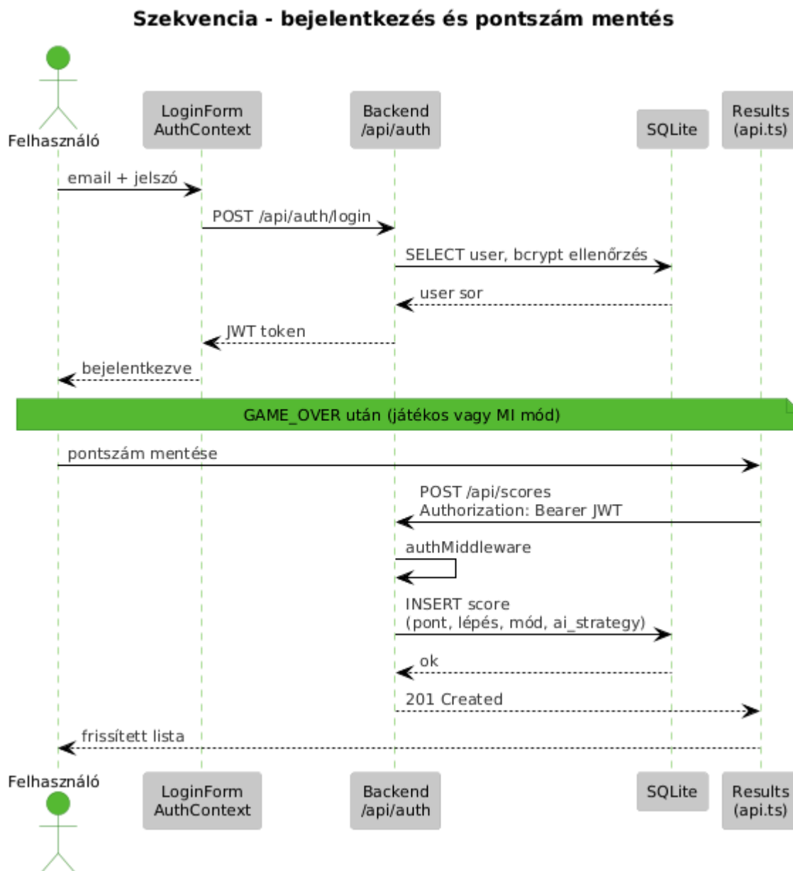
6.9. ábra – Szekvencia: POST /api/auth/login és JWT, majd GAME_OVER után POST /api/scores a tokennel; a backend SQLite -ba ír, a kliens frissített listát kap.
