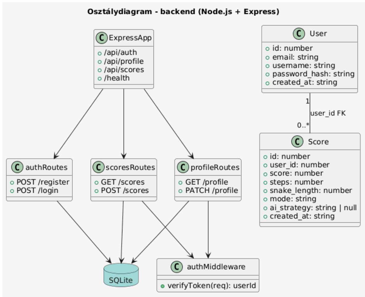
3.3. ábra – Backend osztálydiagram: REST végpontok, JWT middleware, valamint a User–Score kapcsolat az SQLite adatbázissal.
