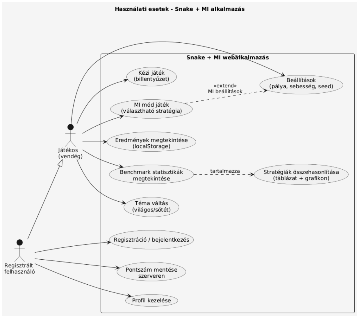
6.0. ábra – Használati esetek: vendég és regisztrált felhasználói szerepkörök, a fő funkciók és az include/extend kapcsolatok.
