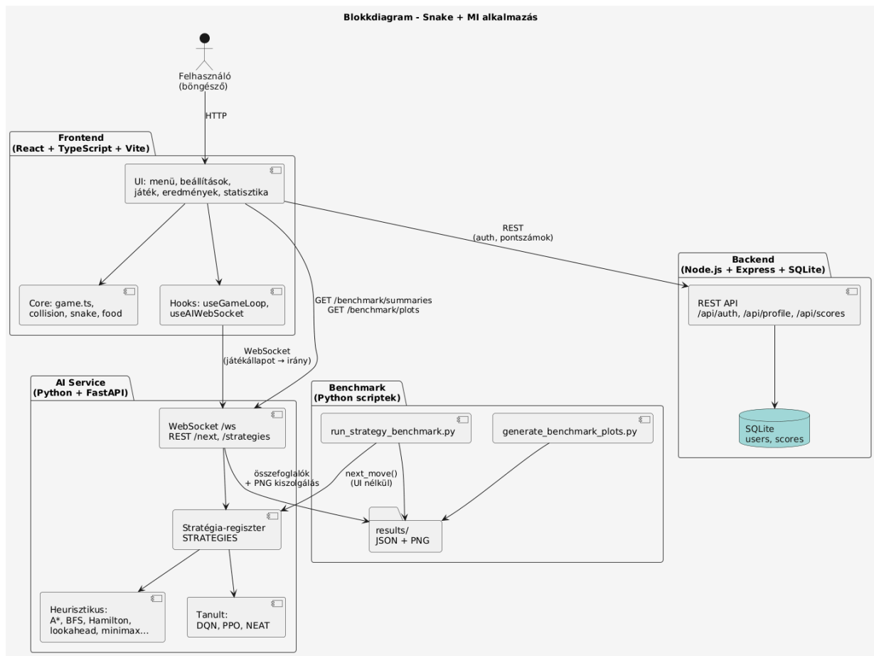
3.1. ábra – Blokkdiagram: a négy fő komponens (frontend, backend, AI service, benchmark) és a REST, WebSocket, illetve fájlrendszer-alapú adatkapcsolatok.
