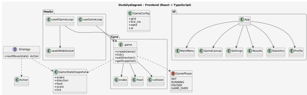
3.2. ábra – Frontend osztálydiagram: a játékmotor (core), a React hookok és a felhasználói felület komponensei közötti függőségek.
