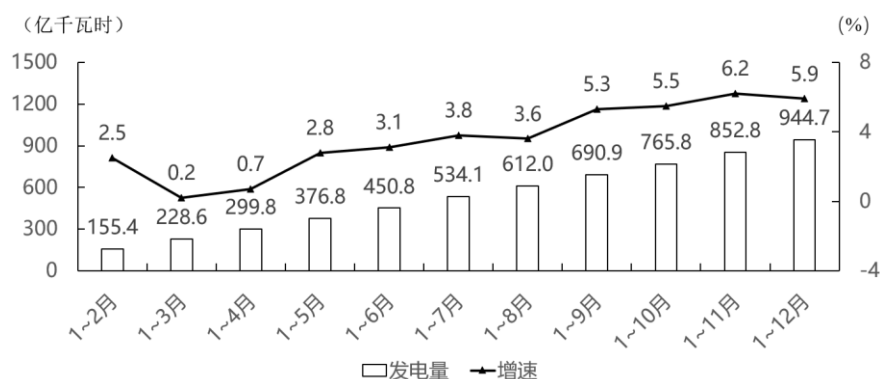
图1 2020年2~12月J省累计发电及同比增速
