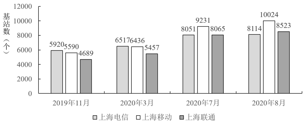
图 上海5G室外基站布局情况
