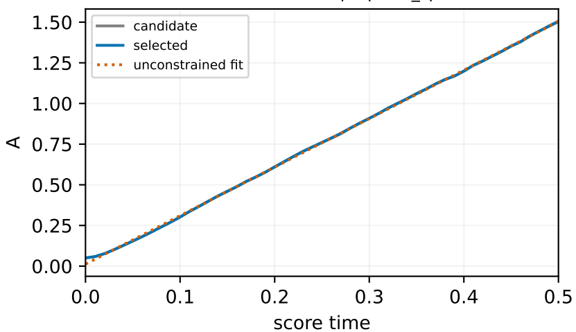
ck2:A:VAL116::NOS::native_velocity_y
