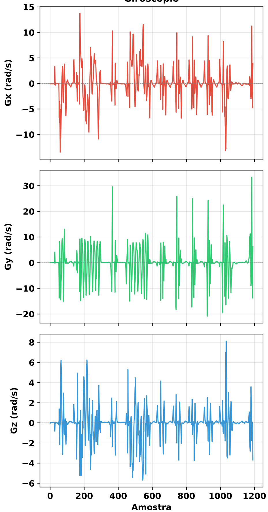
Giroscópio
