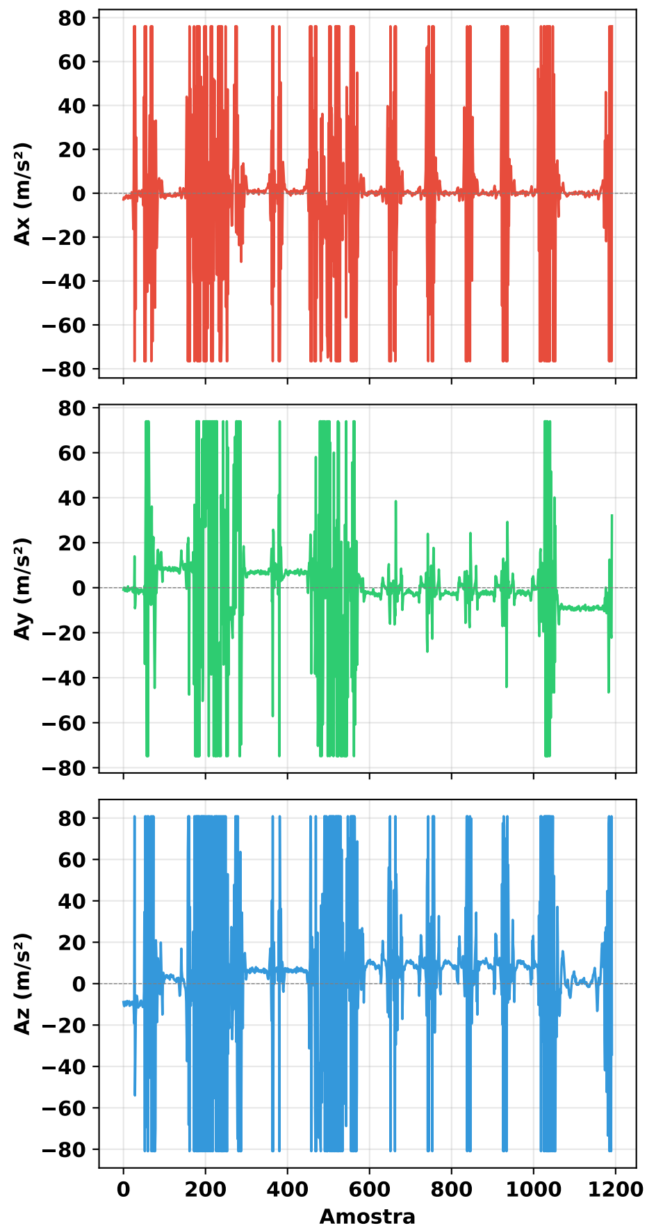
Acelerômetro
