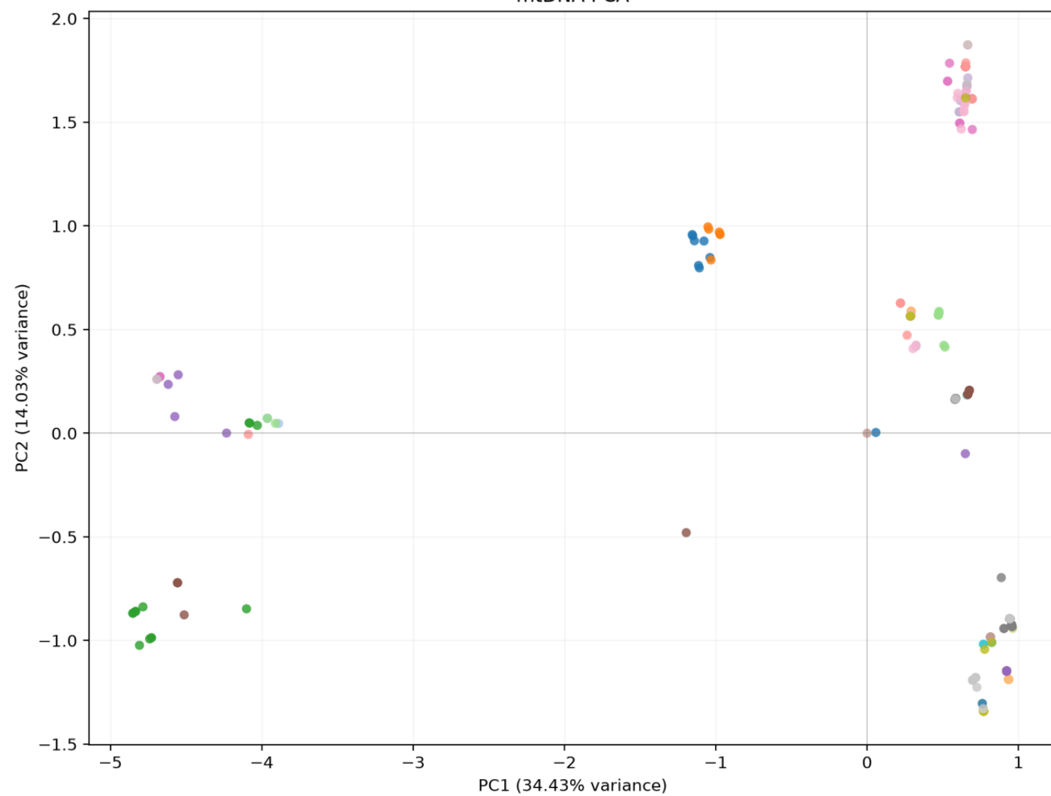
D. mtDNA PCA
