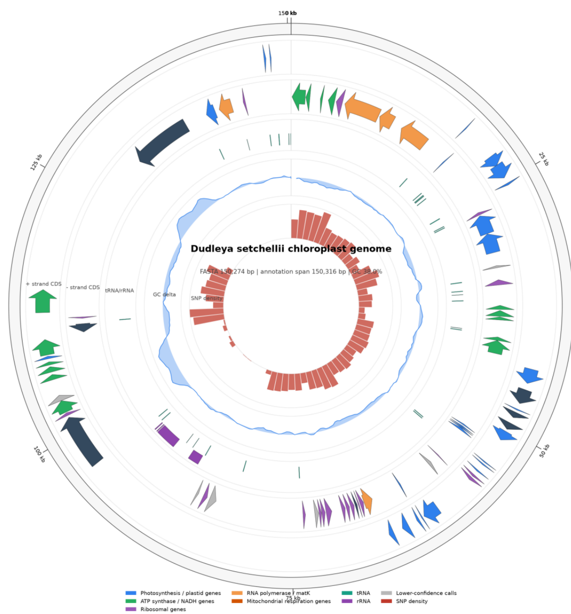
A. cpDNA circular genome map
