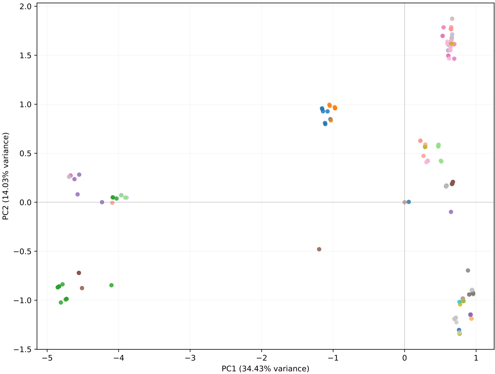
mtDNA PCA
