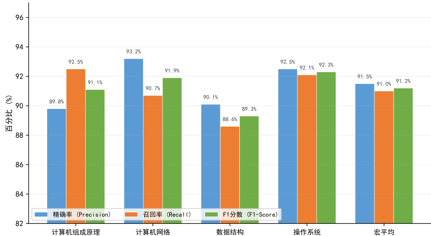
图4.2 逐类别分类性能指标对比
