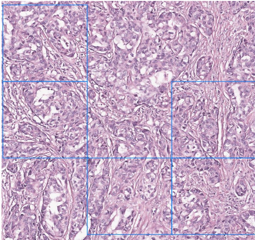
AI 스코어
