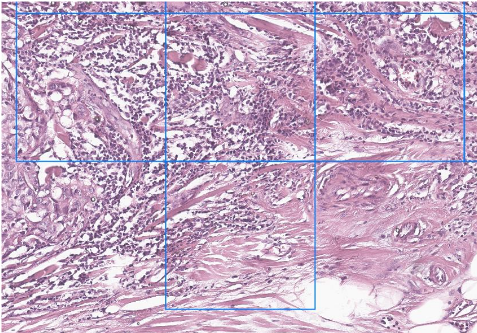
AI 스코어
