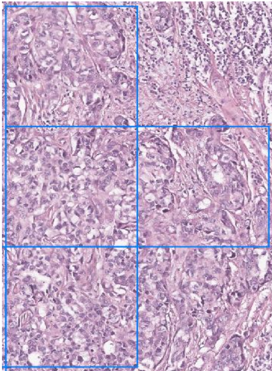
AI 스코어
