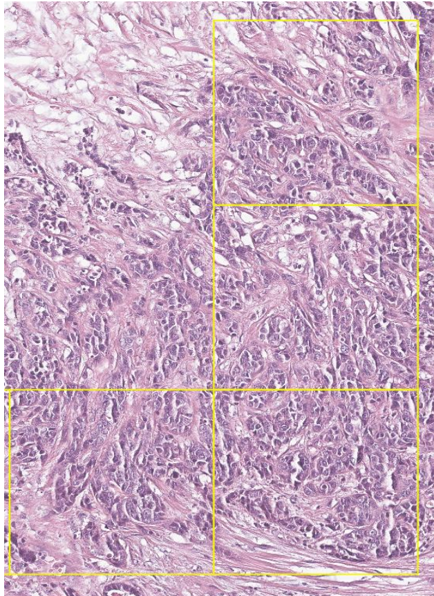
AI 스코어
