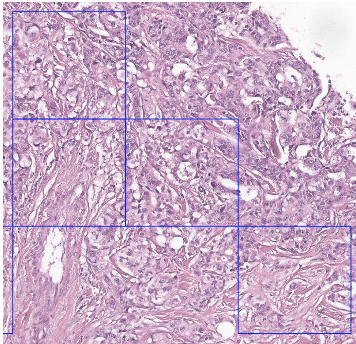
AI 스코어
