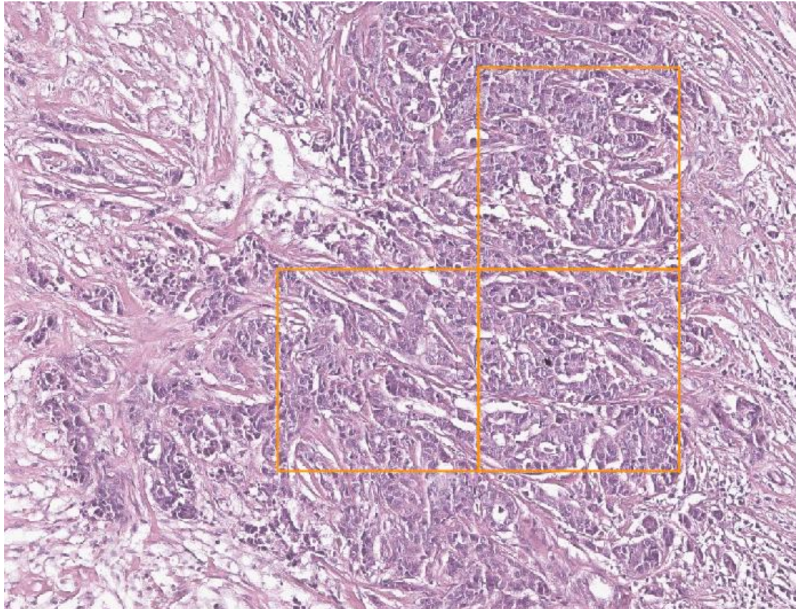
AI 스코어
