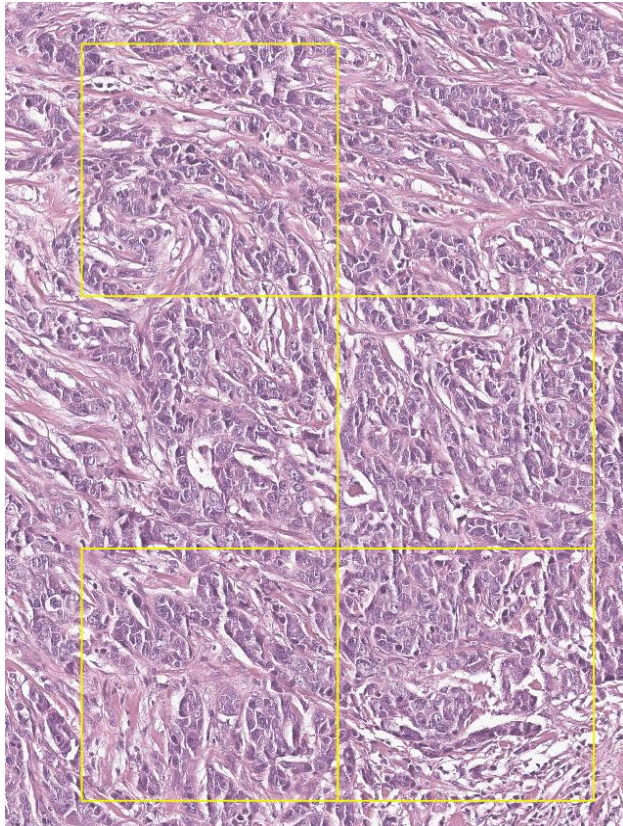
AI 스코어
