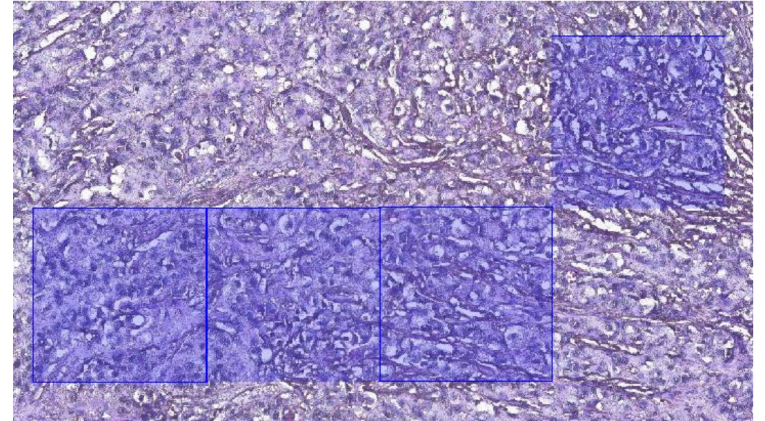
Astromapper 매핑 결과
