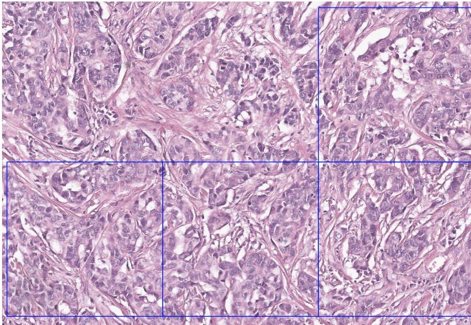
AI 스코어
