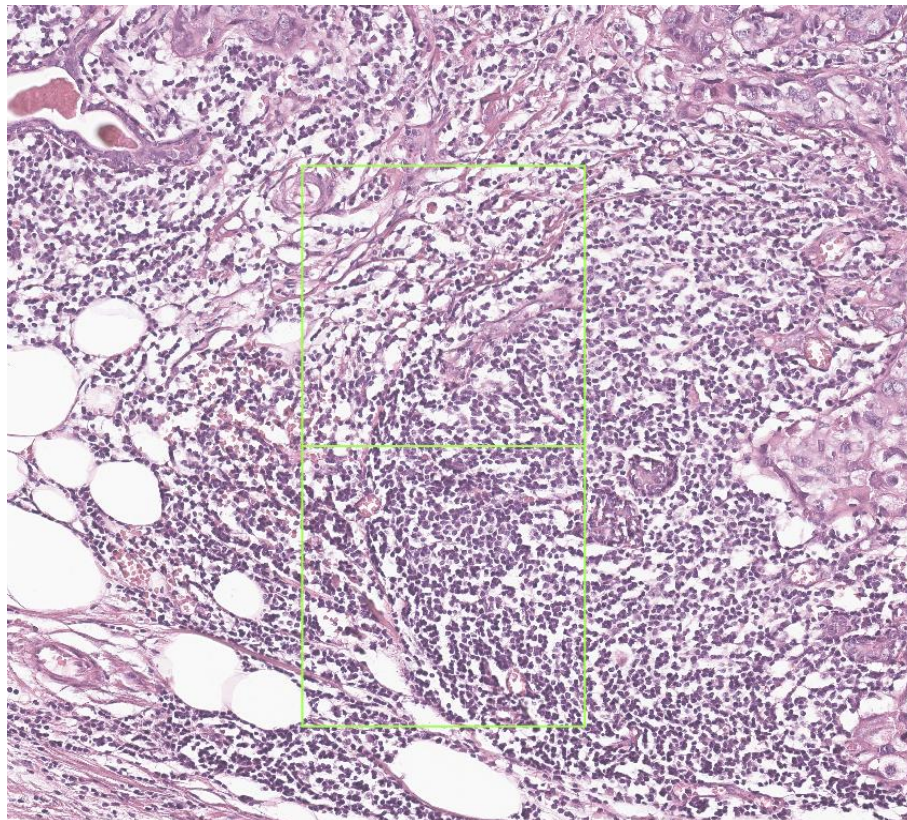
AI 스코어
