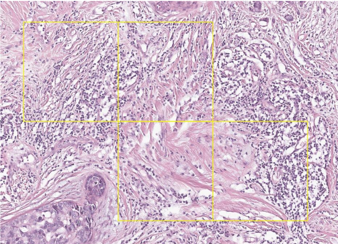
AI 스코어
