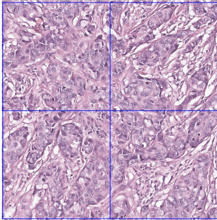
AI 스코어
