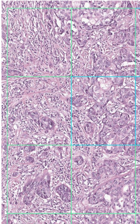
AI 스코어
