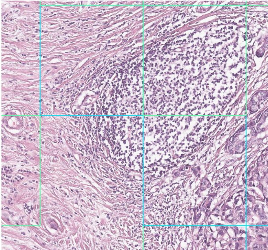
AI 스코어
