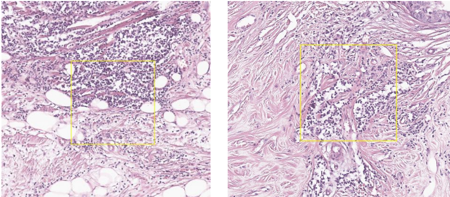
AI 스코어
