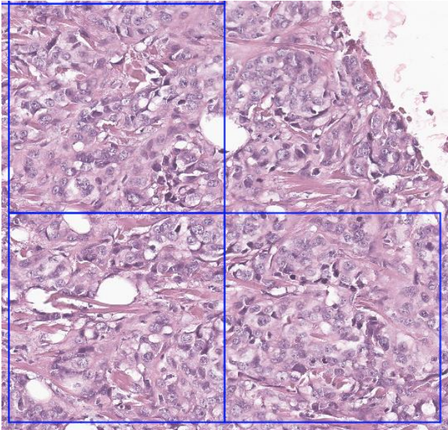
AI 스코어
