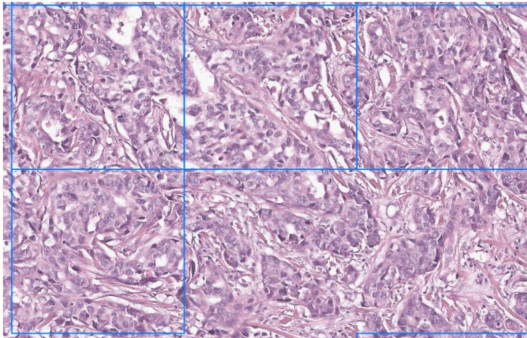
AI 스코어
