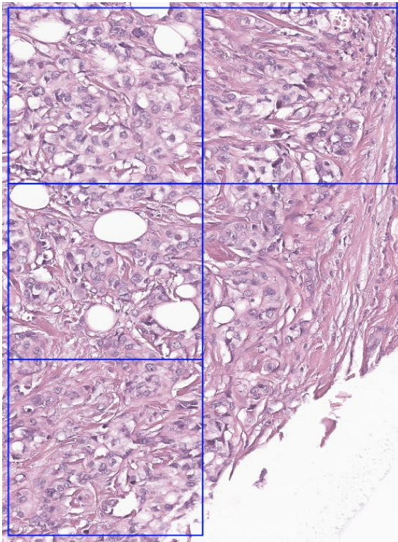
AI 스코어
