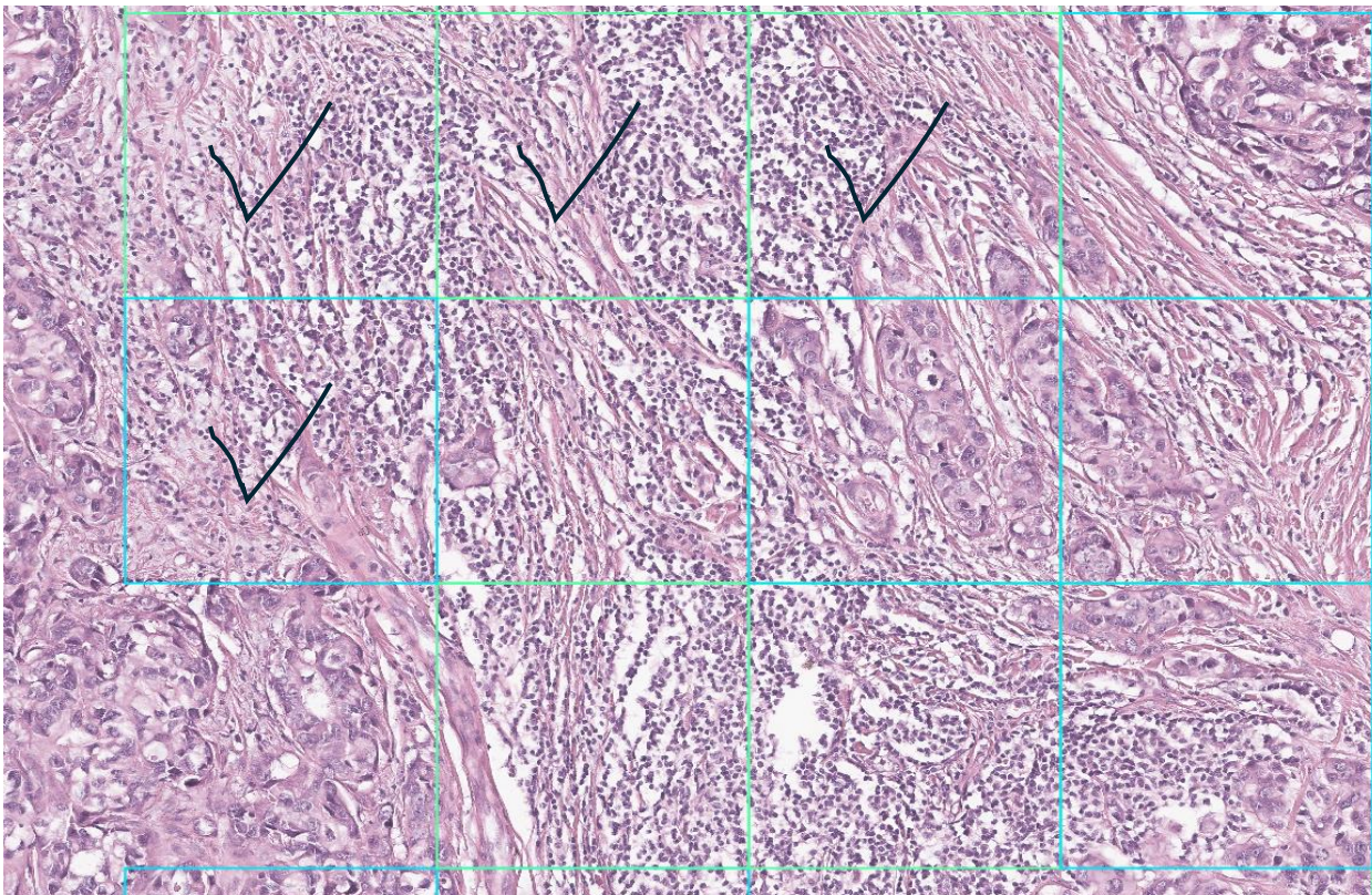
AI 스코어
