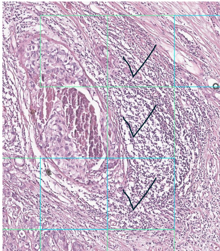
AI 스코어
