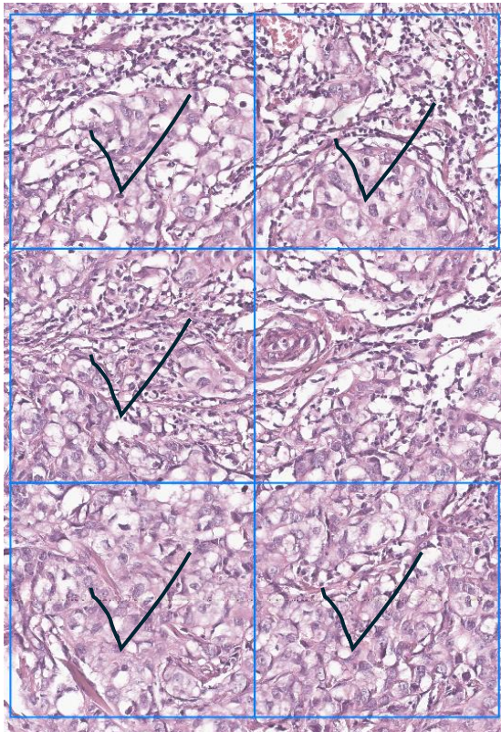
AI 스코어
