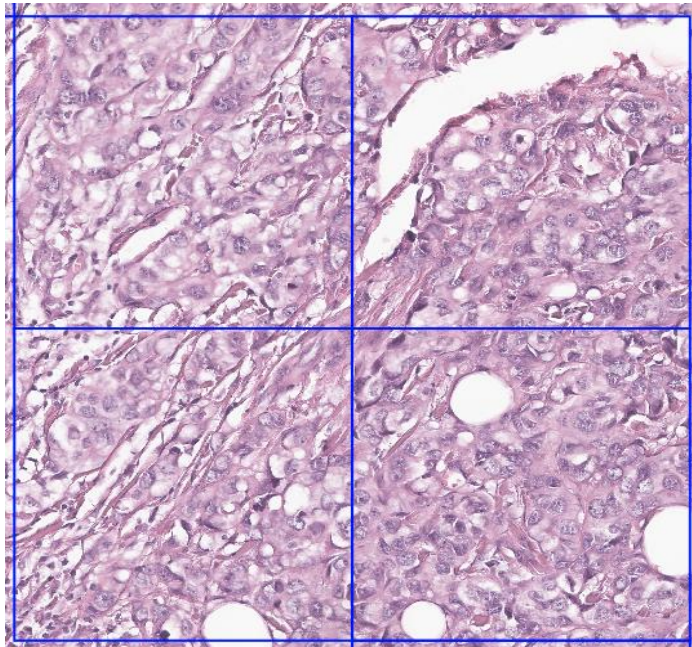
AI 스코어
