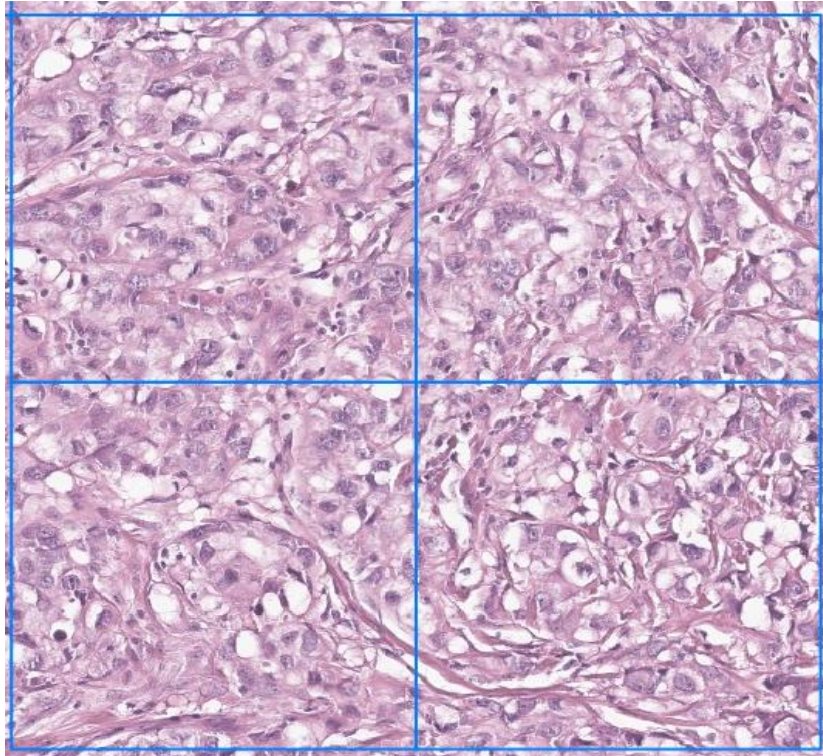
AI 스코어
