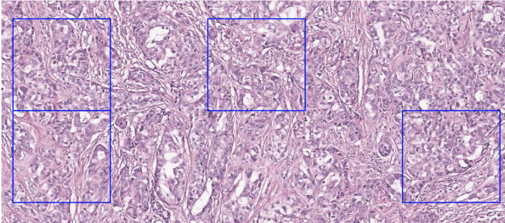
AI 스코어
