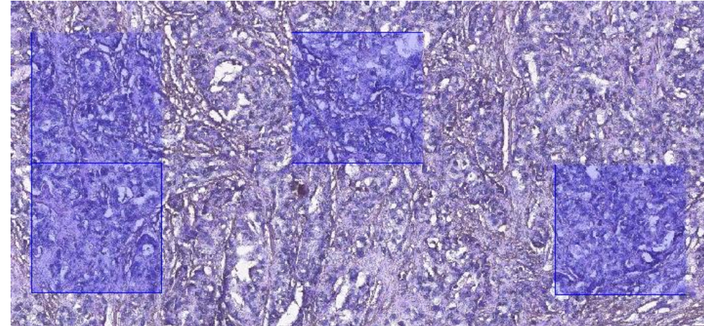
Astromapper 매핑 결과
