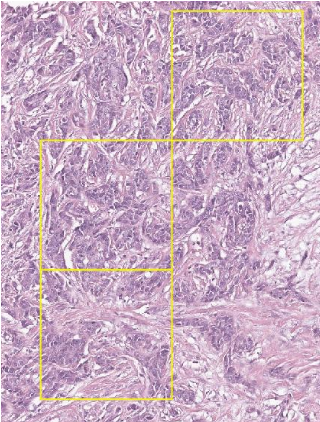
AI 스코어
