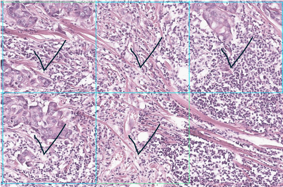
AI 스코어
