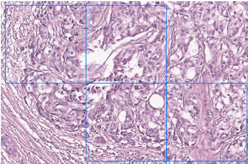
AI 스코어
