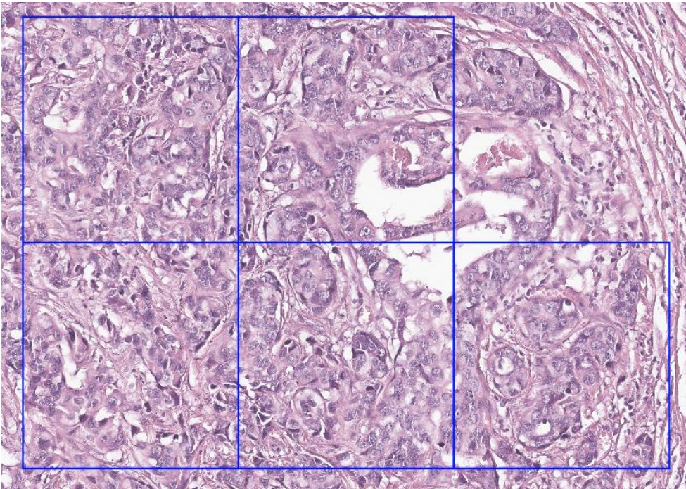
AI 스코어
