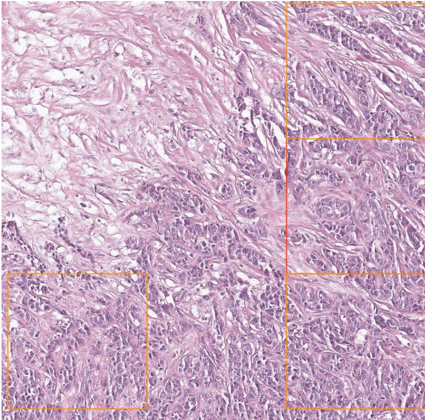
AI 스코어
