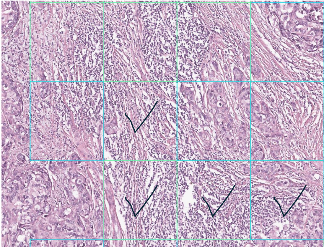
AI 스코어
