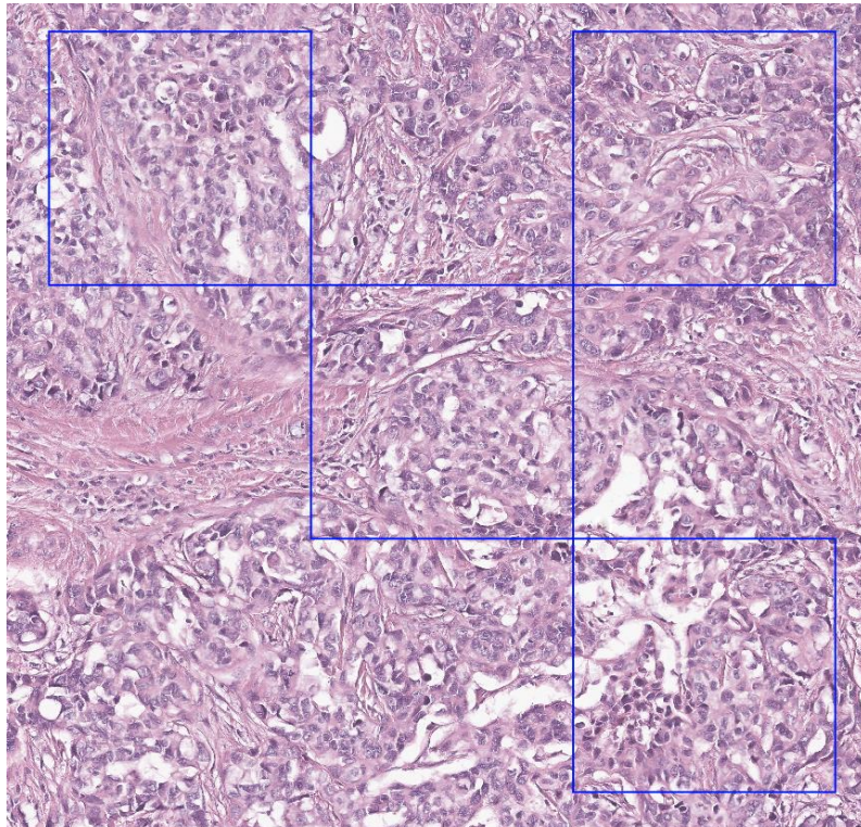
AI 스코어
