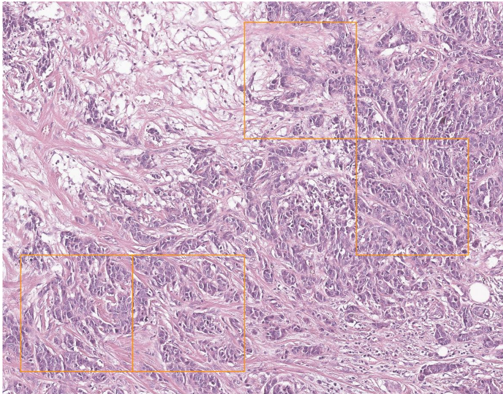
AI 스코어
