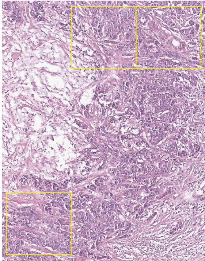
AI 스코어
