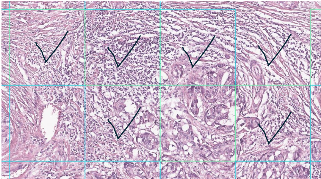
AI 스코어
