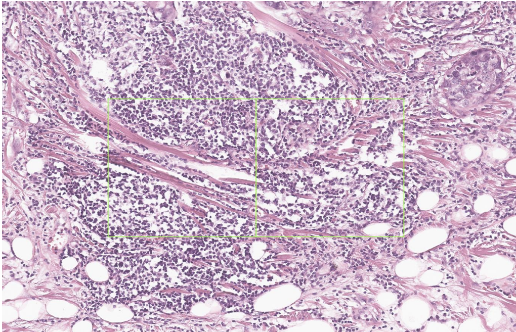
AI 스코어
