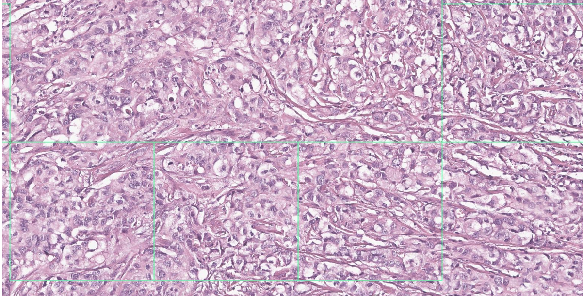
AI 스코어
