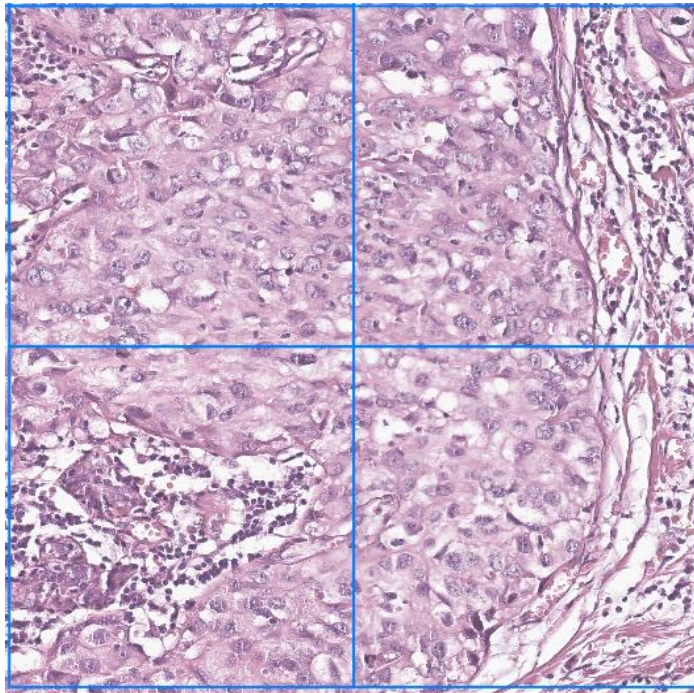
AI 스코어
