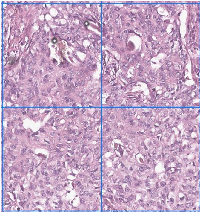
AI 스코어
