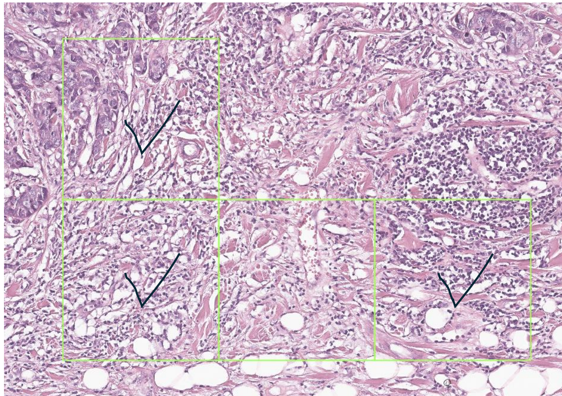
AI 스코어
