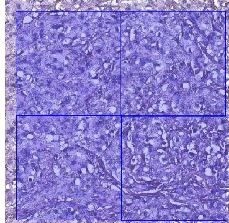
Astromapper 매핑 결과
