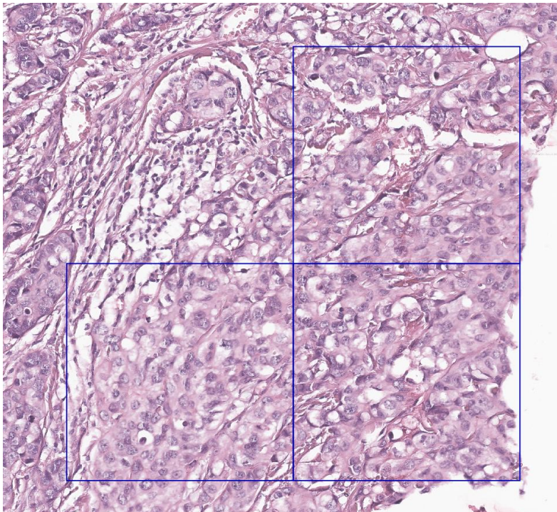
AI 스코어
