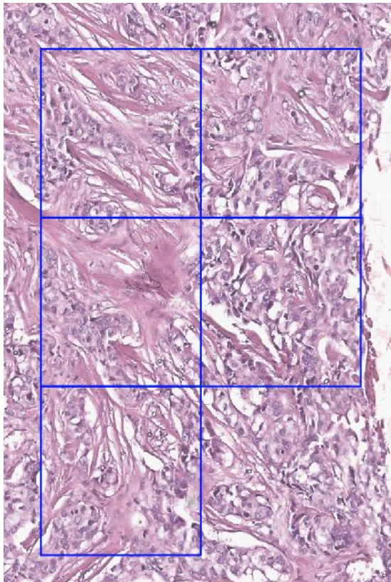
AI 스코어
