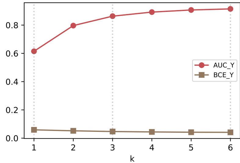
Y reconstruction vs k (Bernoulli Y)
