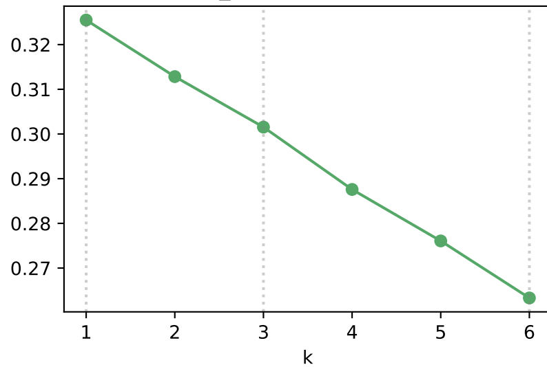
BCE_X vs k (Bernoulli X)
