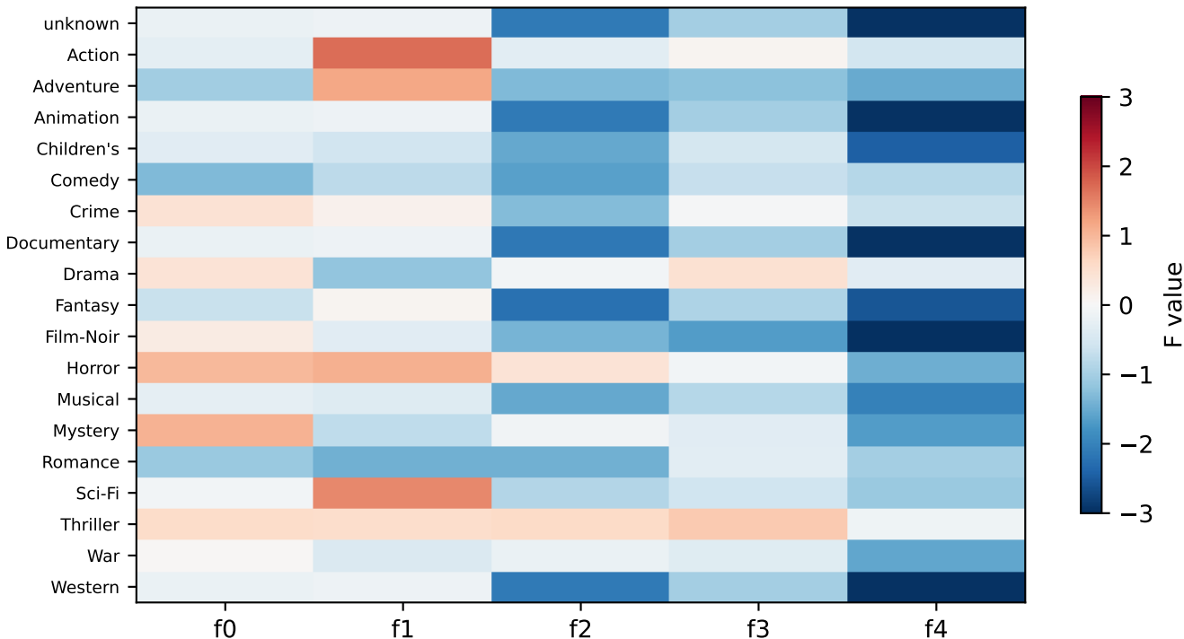
movielens F heatmap (k=5, best trial=0, BIC=28682.2)
