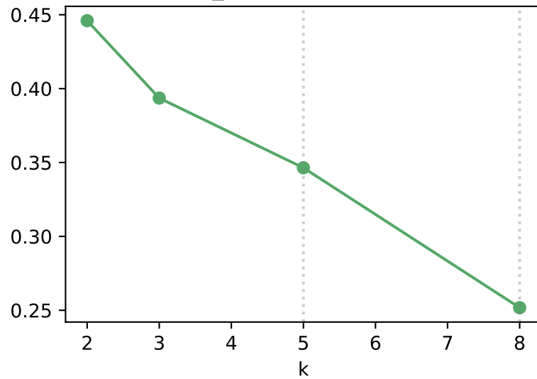
BCE_X vs k (Bernoulli X)
