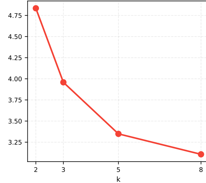
RMSE_Y
