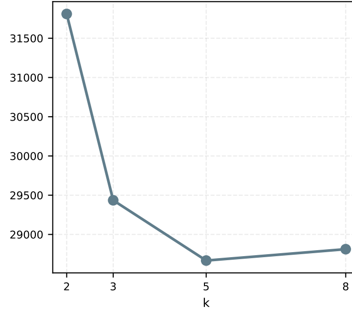
BIC
