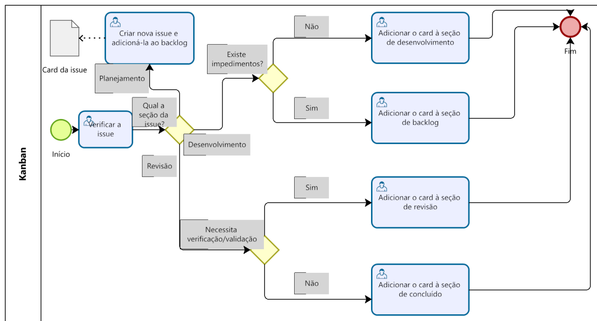
Figura 8 – BPMN Kanban
