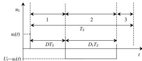
图 A2 横/纵坐标为非定量的、简单标目的函数图形
