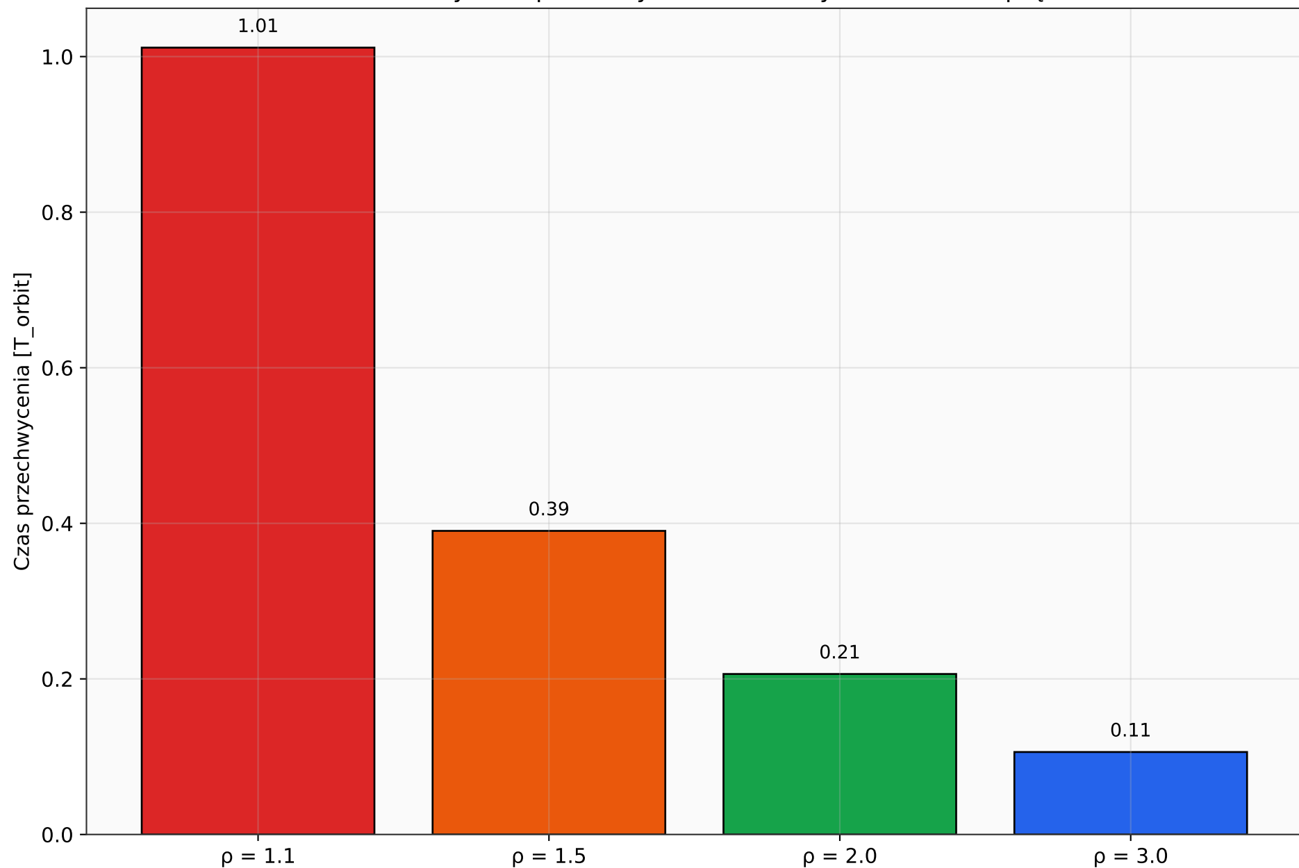
Znormalizowany czas przechwycenia dla różnych stosunków prędkości
