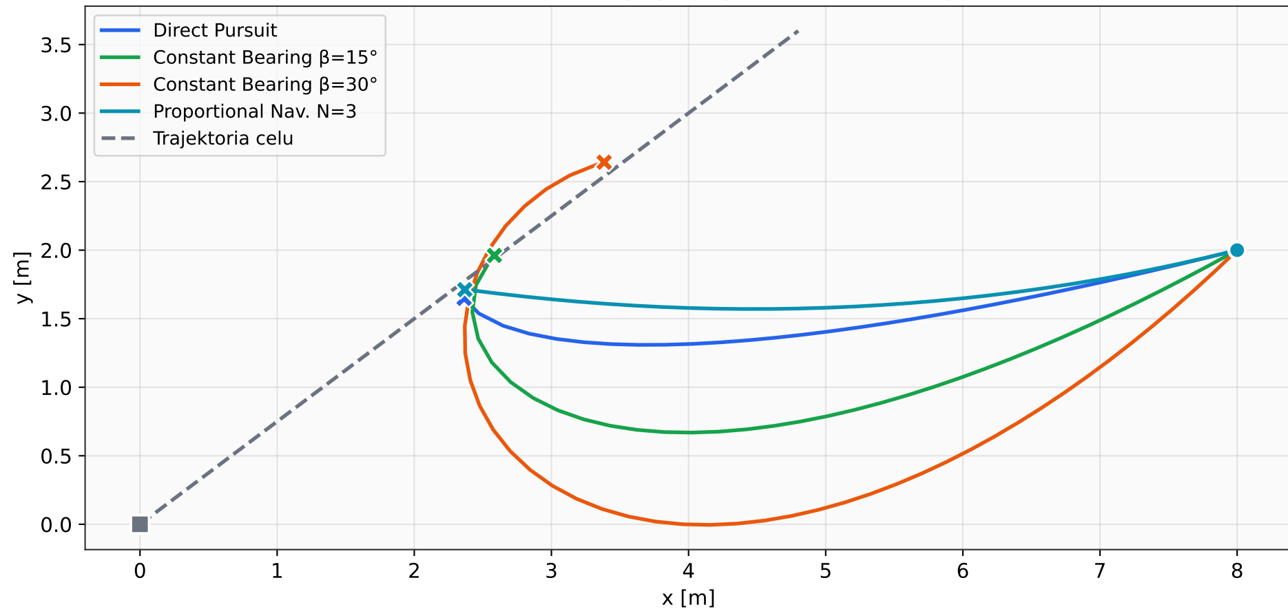
Porównanie strategii pościgu dla celu liniowego
