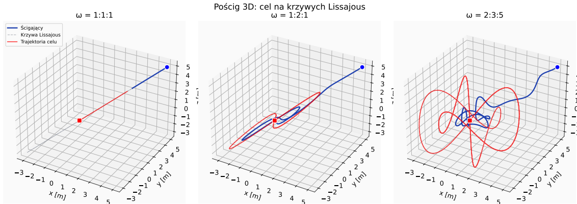
Rysunek 8: Pościg 3D dla celu na krzywych Lissajous o różnych stosunkach częstotliwości \omega_x : \omega_y : \omega_z . Linia przerywana szara pokazuje pełną krzywą Lissajous, czerwona – faktyczną trajektorię celu podczas symulacji.
