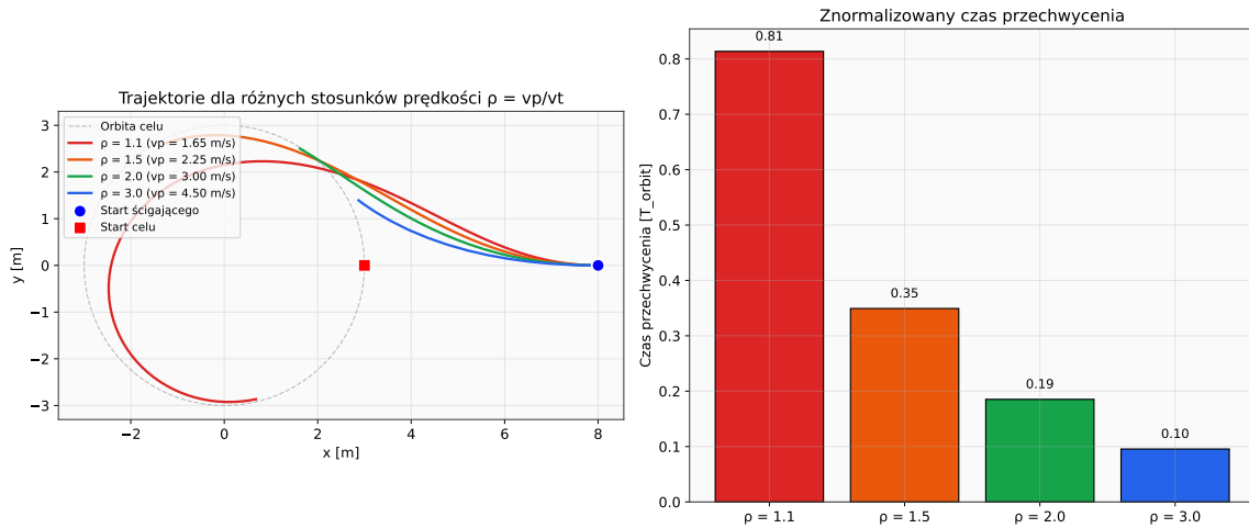
Rysunek 5: Analiza wpływu stosunku prędkości \rho = v_p/v_t na trajektorię pościgu (lewo) oraz znormalizowany czas przechwycenia (prawo).
