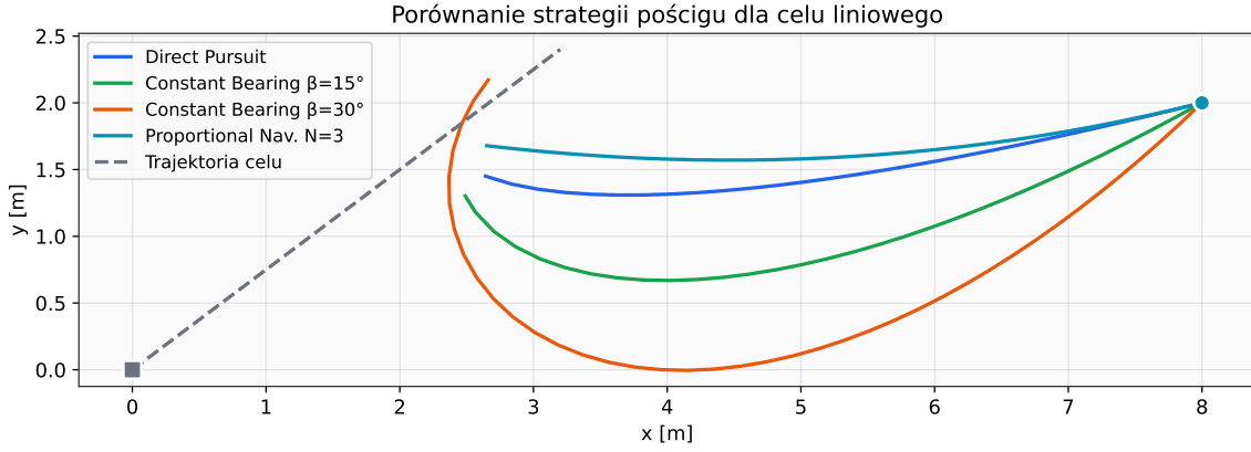
Rysunek 2: Porównanie trajektorii dla różnych strategii pościgu przy celu poruszającym się liniowo. Punkty oznaczają pozycje startowe.
