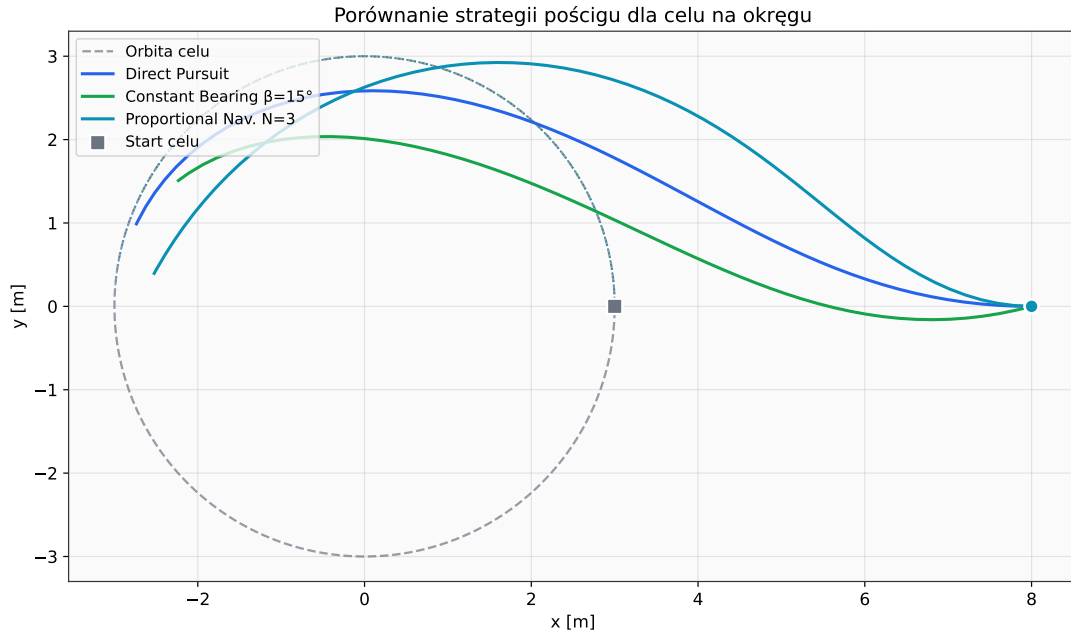
Rysunek 1: Porównanie strategii pościgu dla celu poruszającego się po okręgu. Linia przerywana oznacza orbitę celu.
