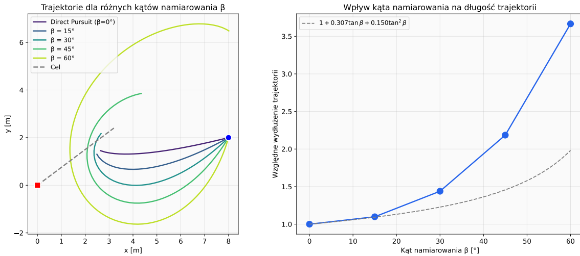
Rysunek 3: Wpływ kąta namiarowania \beta na trajektorię (lewo) oraz względne wydłużenie trajektorii w funkcji kąta (prawo). Linia przerywana pokazuje dopasowanie analityczne.
