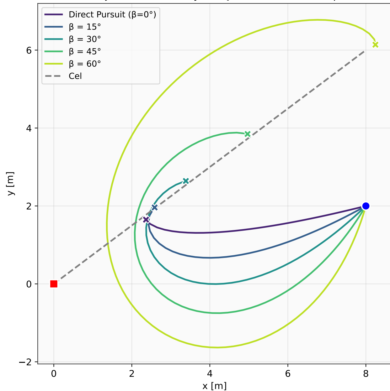
Trajektorie dla różnych kątów namiarowania \beta
