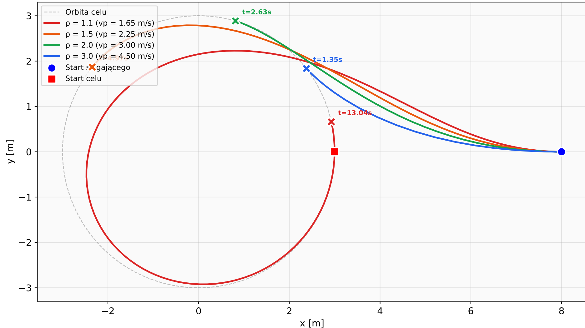
Trajektorie dla różnych stosunków prędkości \rho = v_p/v_t
