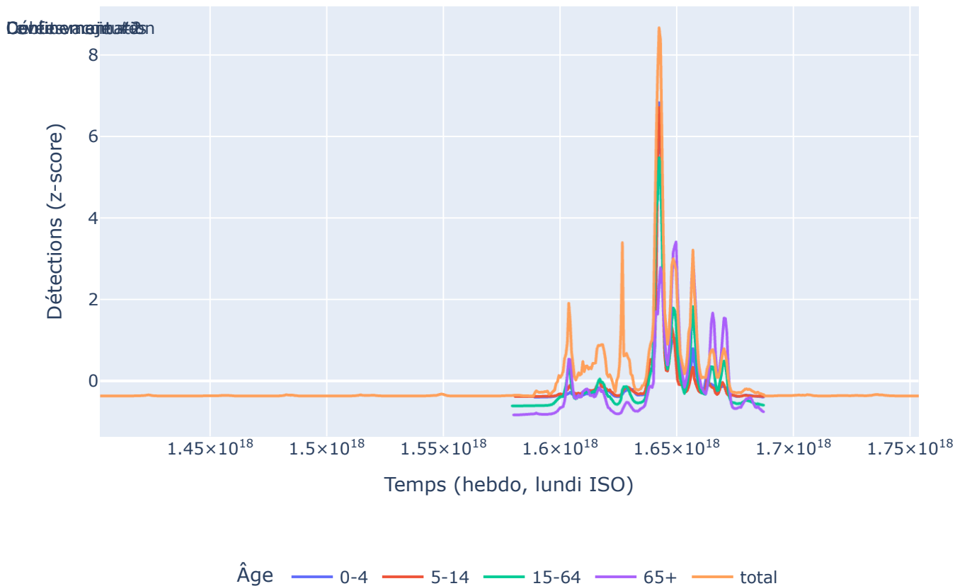
Figure 4 — ERVISS RSV par âge : détections (z-score)
