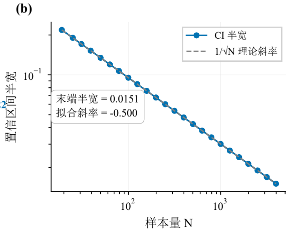
导通概率估计收敛：N = 3981 时 CI 半宽 0.015，误差按 1/\sqrt{N} 收缩
