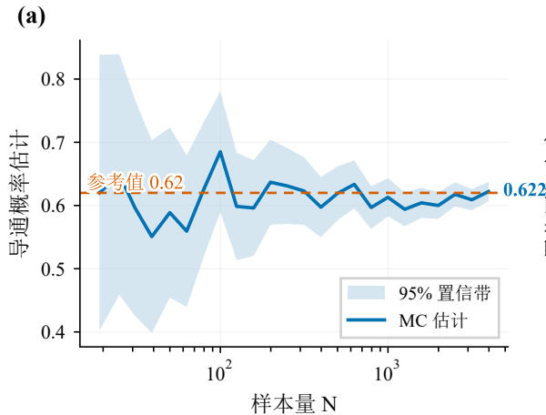
导通概率估计收敛：N = 3981 时 CI 半宽 0.015，误差按 1/\sqrt{N} 收缩
