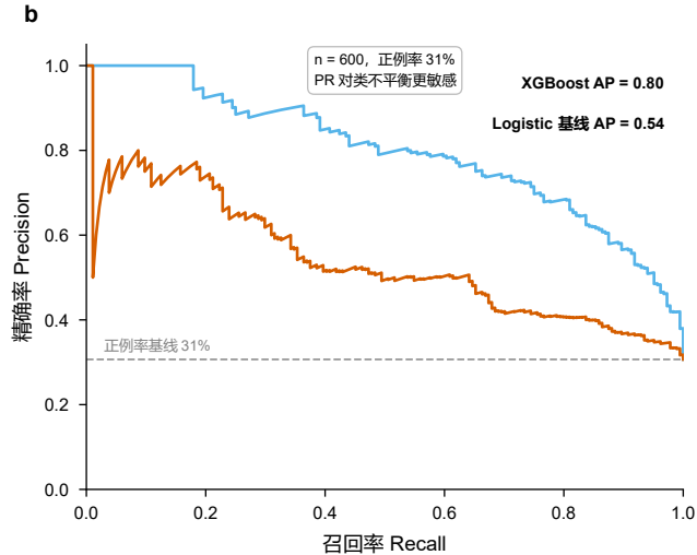
XGBoost AUC 0.89 / AP 0.80, 全阈值段优于 Logistic 基线
