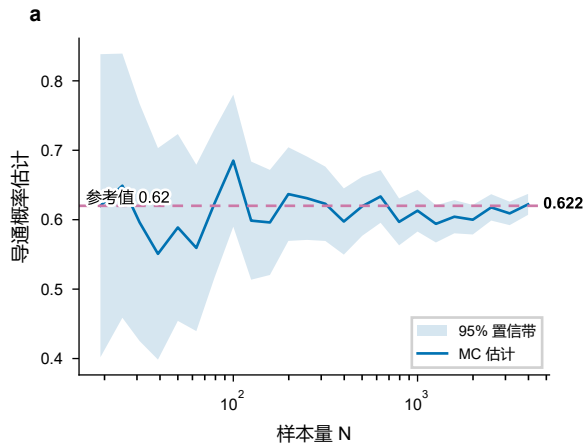
导通概率估计收敛: N = 3981 时 CI 半宽 0.015, 误差按 1/\sqrt{N} 收缩
