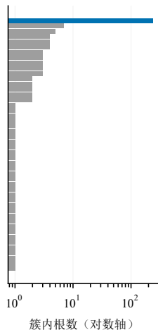
簇尺寸谱（48 簇）
