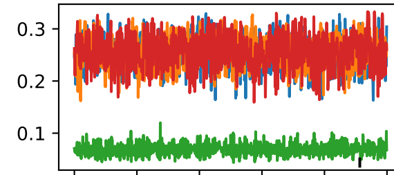
f_auto Draw
