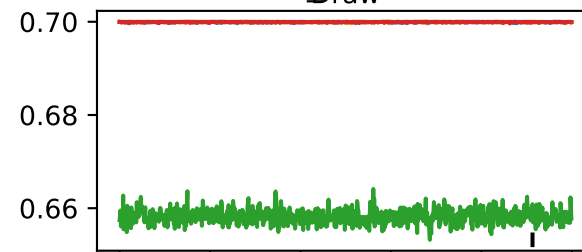
f_auto Draw
