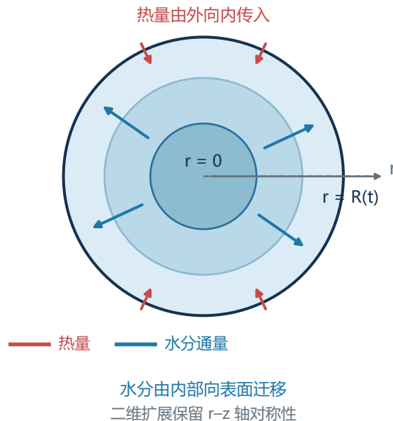
(b) 轴对称径向模型
