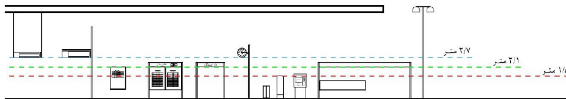
شکل ۷-۴ ارتفاع مجاز نصب تابلوها در ایستگاه شبکه حمل و نقل ریلی شهری و حومه
